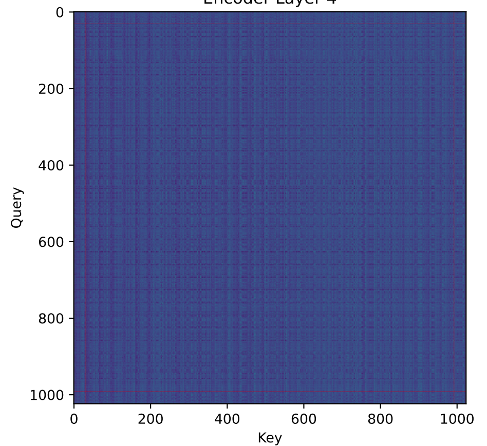
Encoder Layer 4
