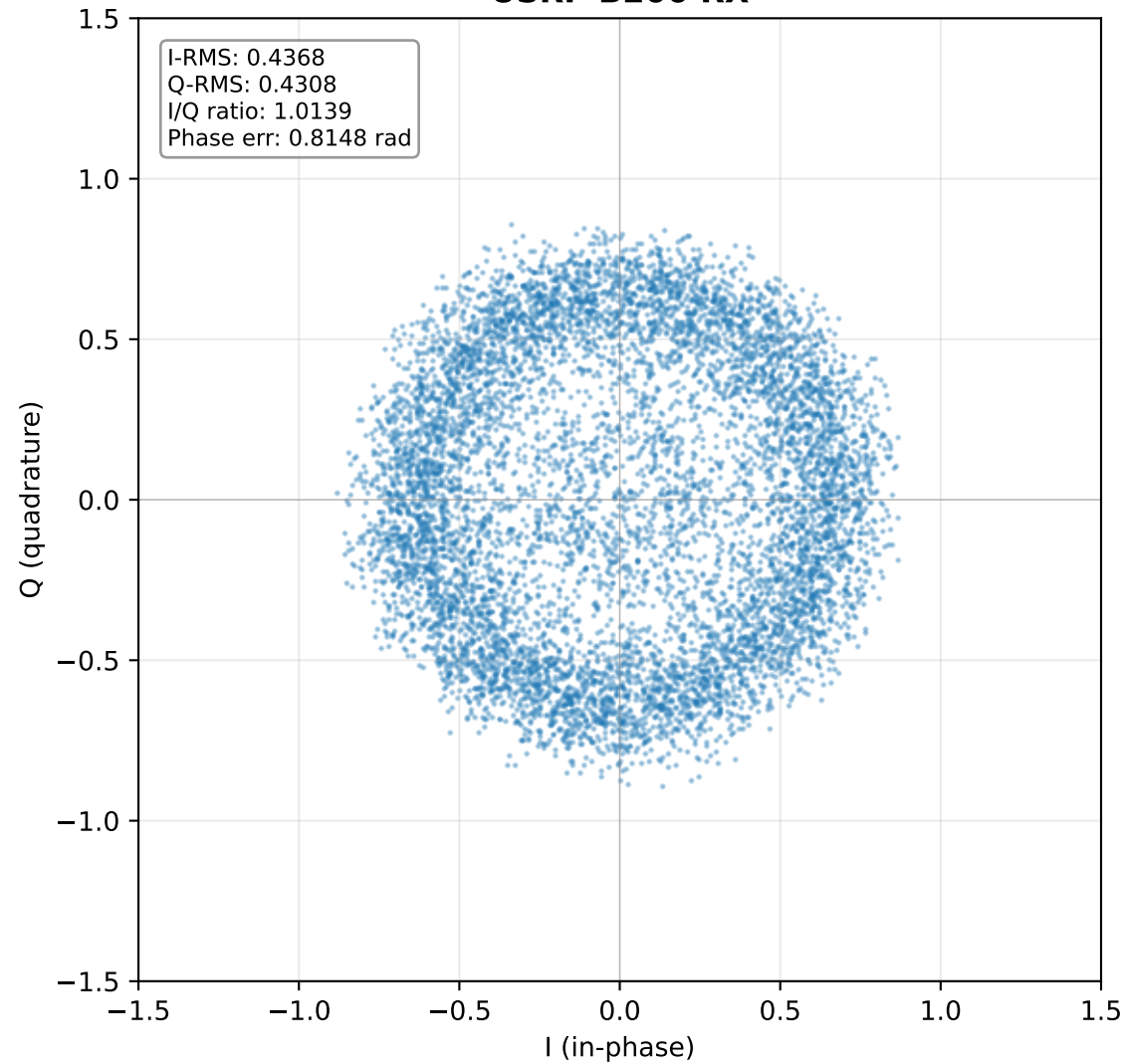
USRP B200 RX
