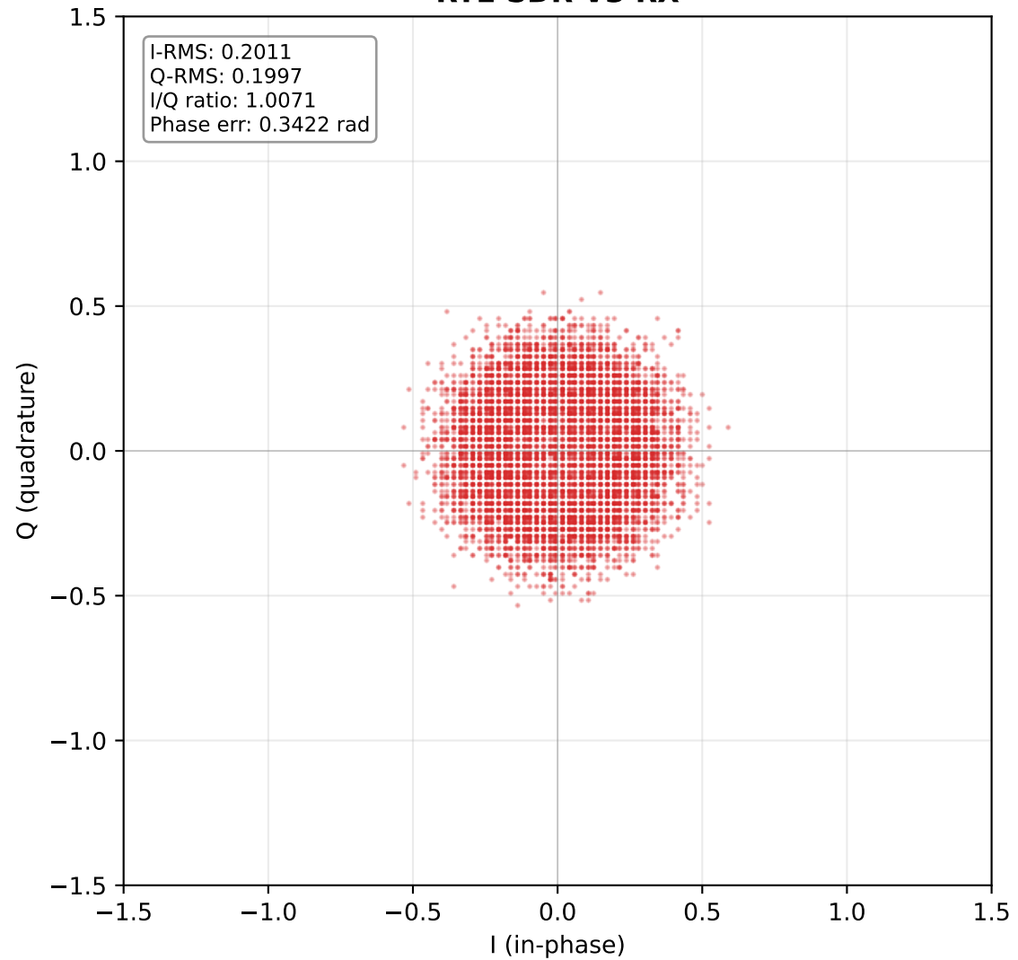
RTL-SDR V3 RX
