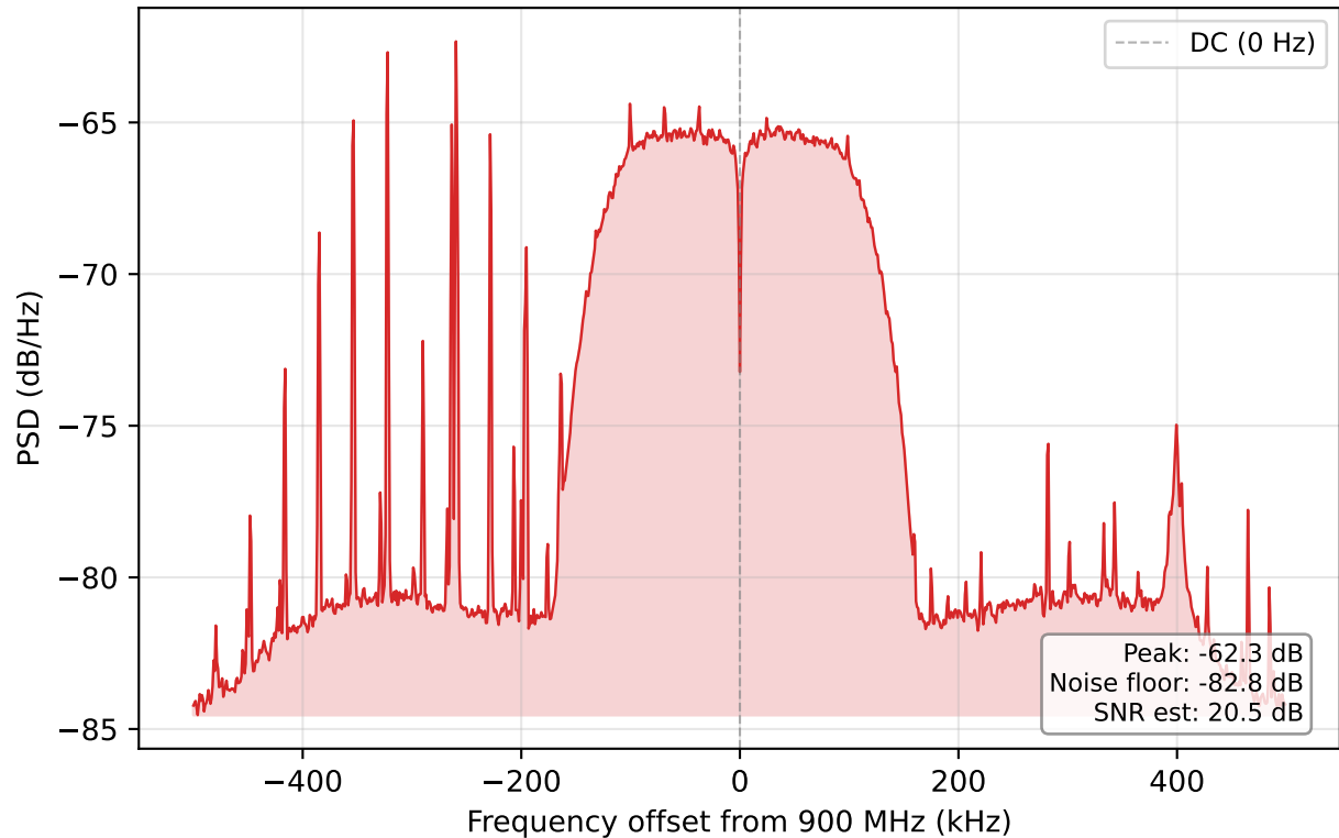
RTL-SDR V3 RX
