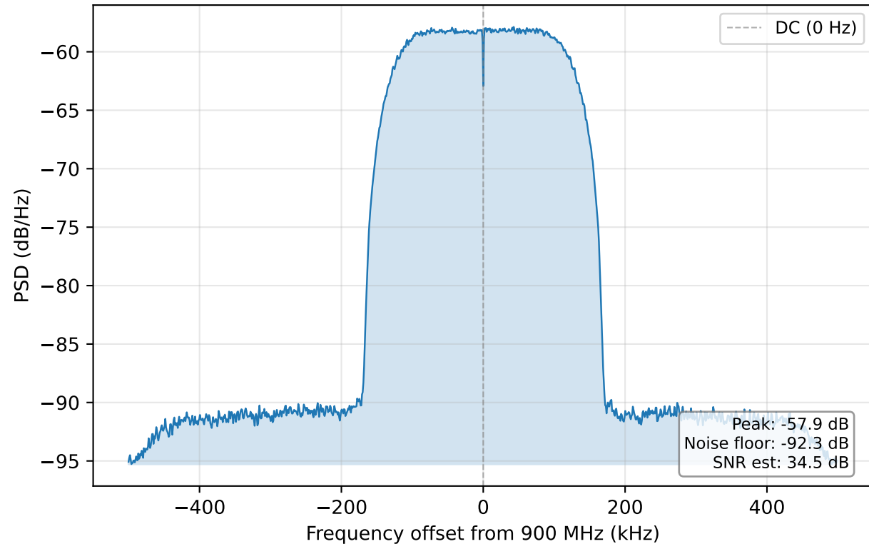
USRP B200 RX
