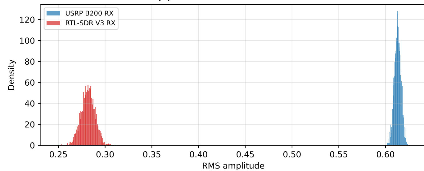
(d) RMS distribution KS=1.0000
