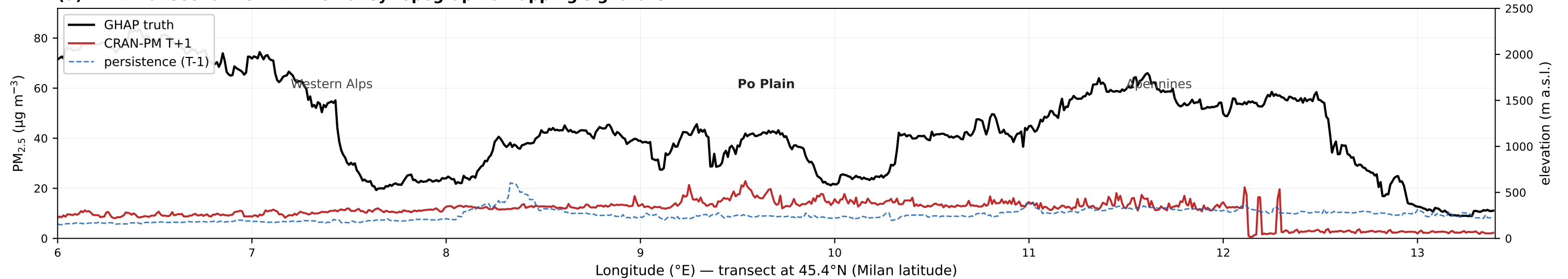
(d) W→E transect at 45.4°N : Po Valley topographic trapping signature
