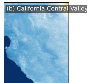
GT (zoom)
