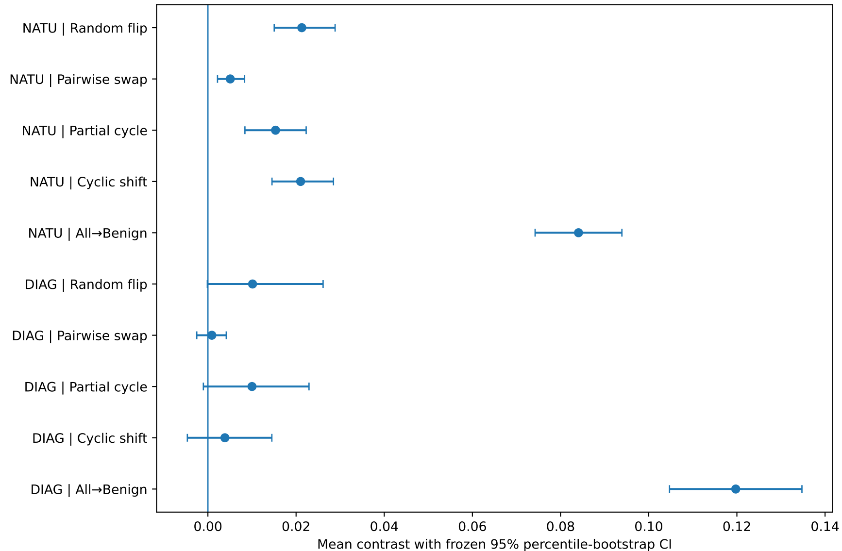
Macro F1 — Round 8
