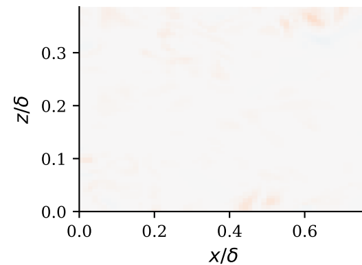
(d) Canonical WALE
