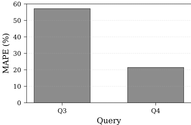
MAPE - Abacus
