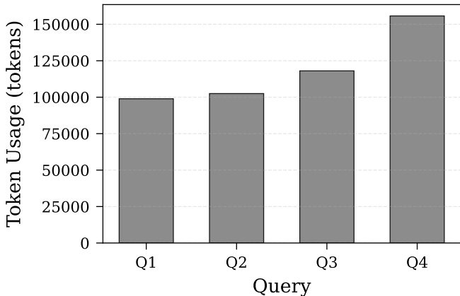
Token Usage - Abacus
