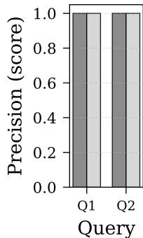
Precision
