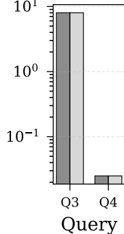
Absolute Error
