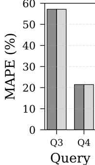
MAPE
