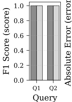
F1 Score
