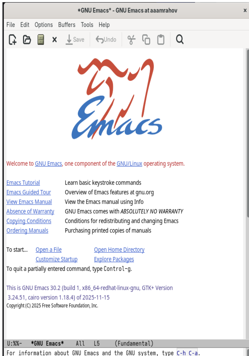
Рисунок 2.1: Запуск Emacs
