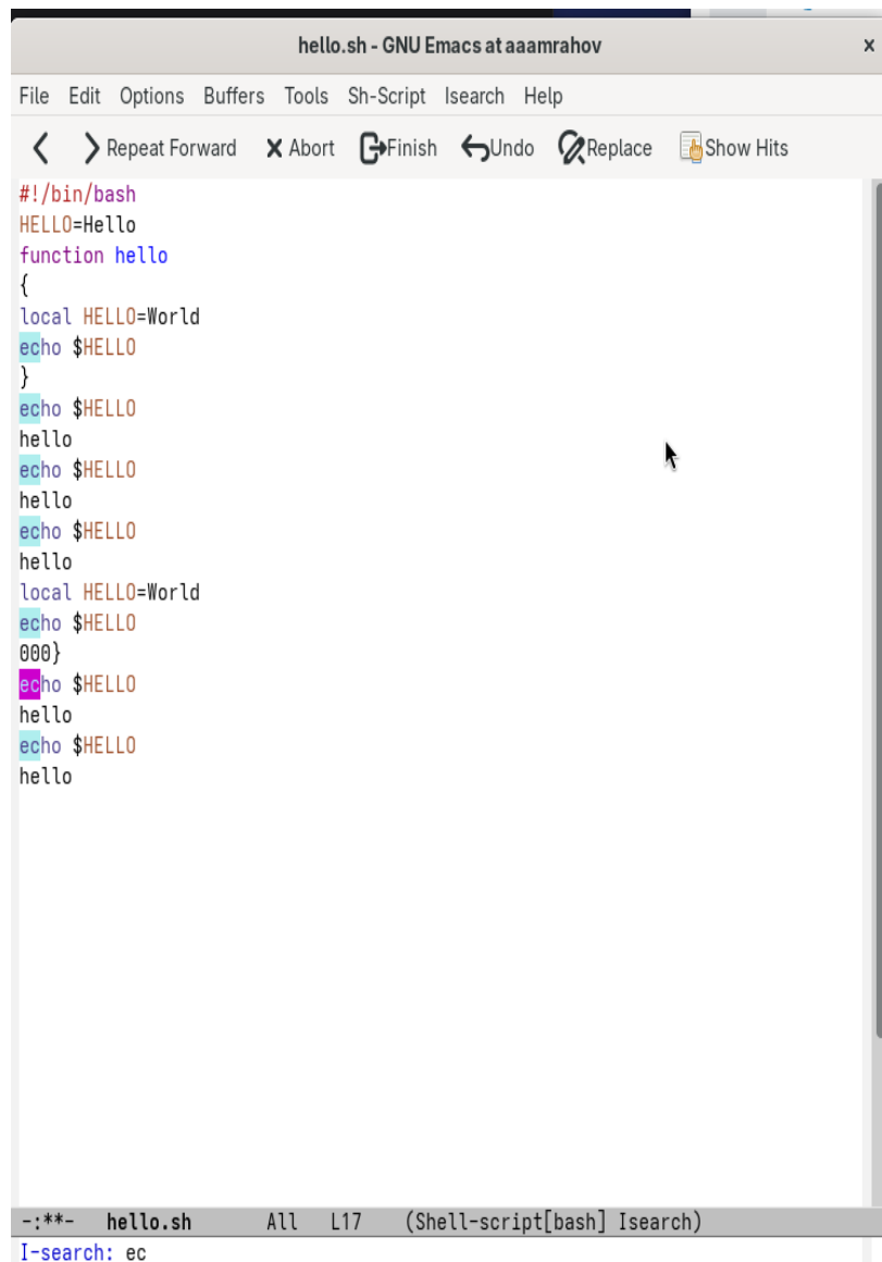
Рисунок 2.12: Режим поиска
