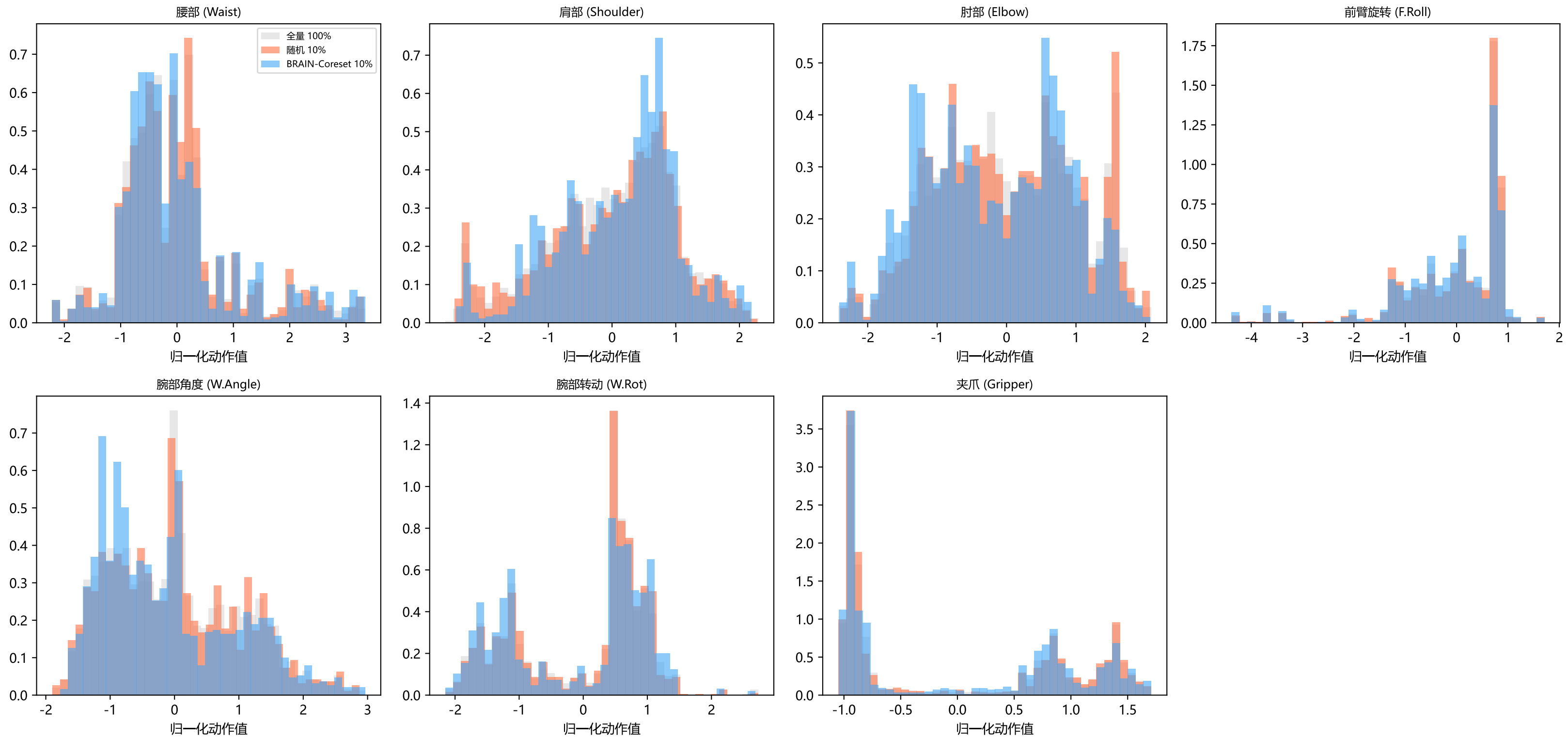
图 4: 动作各维度分布 — 全量数据 vs 随机 10% vs BRAIN-Coreset 10%
