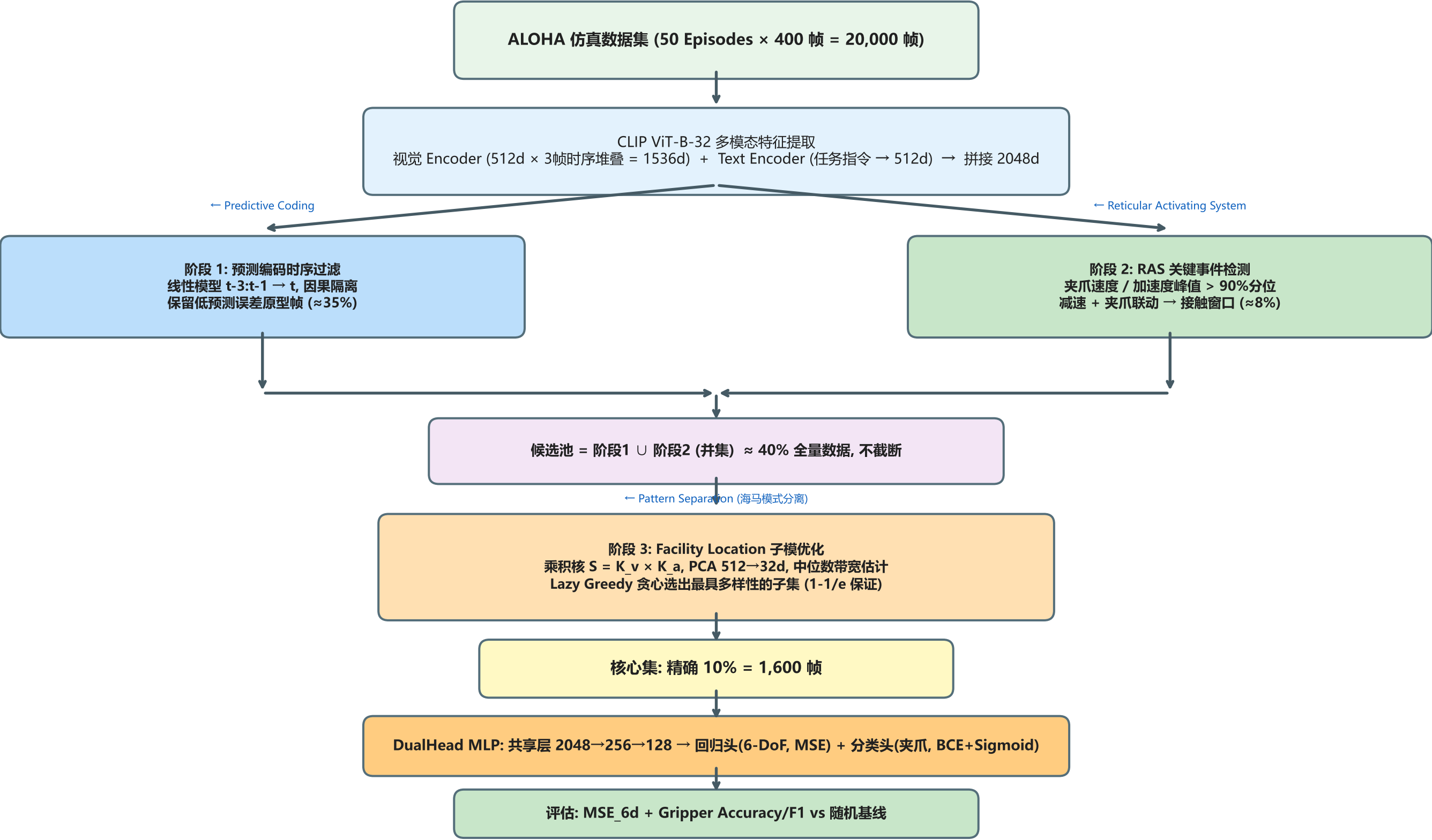
图 1: BRAIN-Coreset VLA 算法框架流程图
