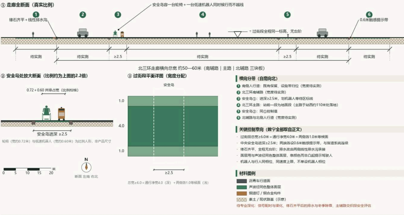
断面 DZS-1 · 声波径穿越城市道路（概念断面示意）
