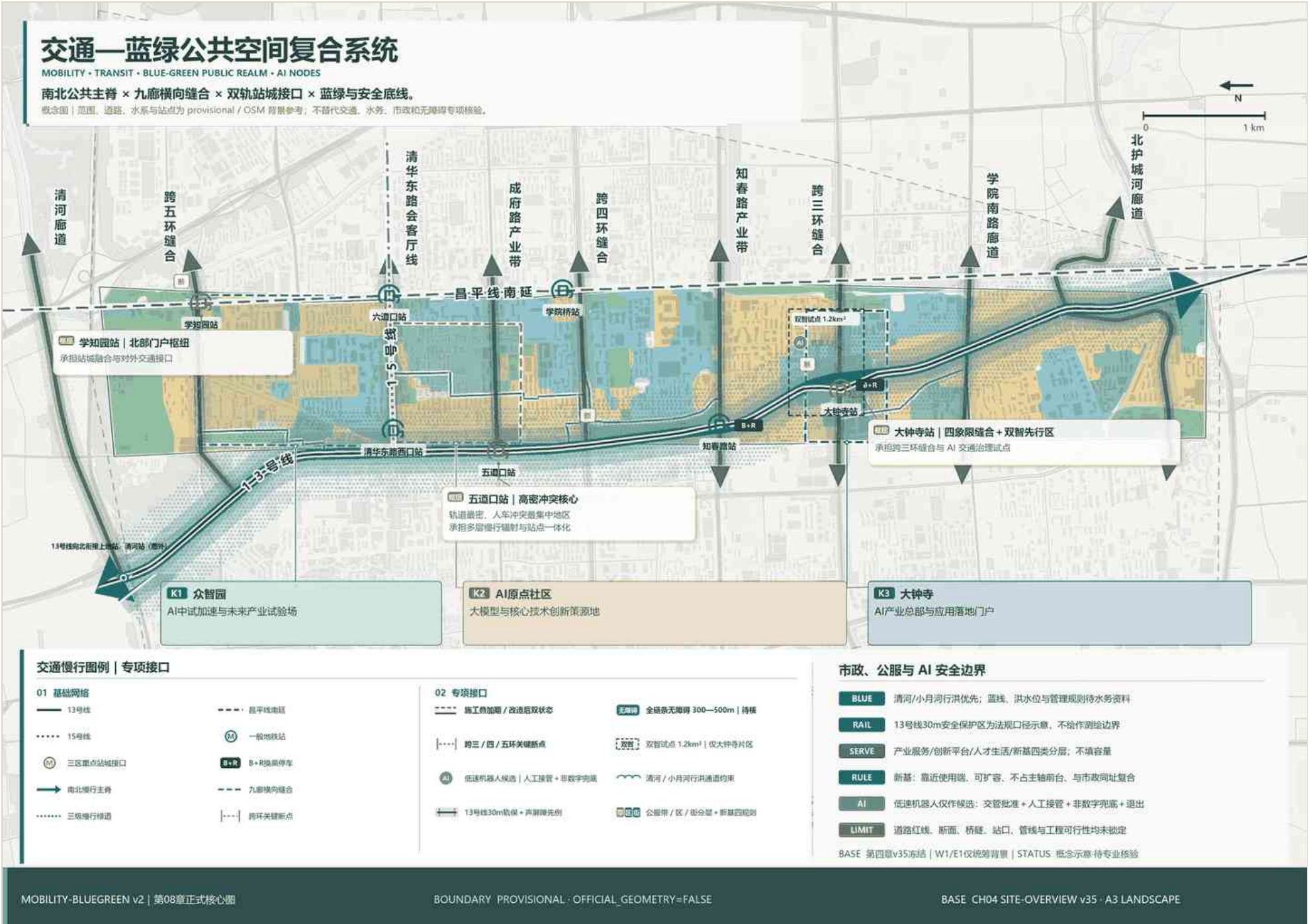
图8-1 | 交通慢行、轨道接驳、蓝绿公共空间与AI场景节点复合系统。综合表达交通慢行、轨道接驳、蓝绿公共空间与 AI 场景节点关系；线位、容量、权属和工程条件仍待正式资料与专业校核。[source:CH8-TRANSPORT]
