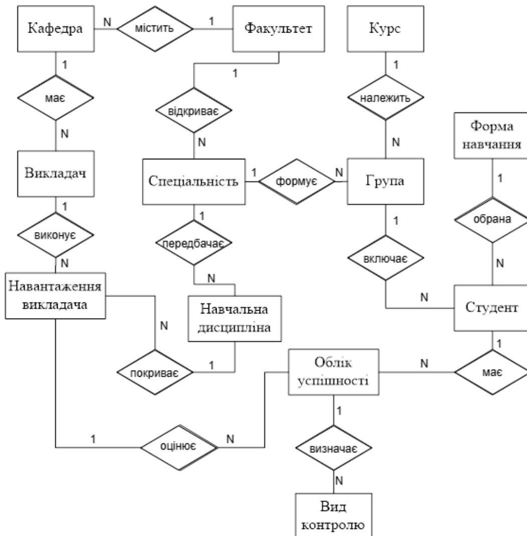
Рисунок 1.1 – ER-діаграма предметної області «Деканат ВНЗ»
