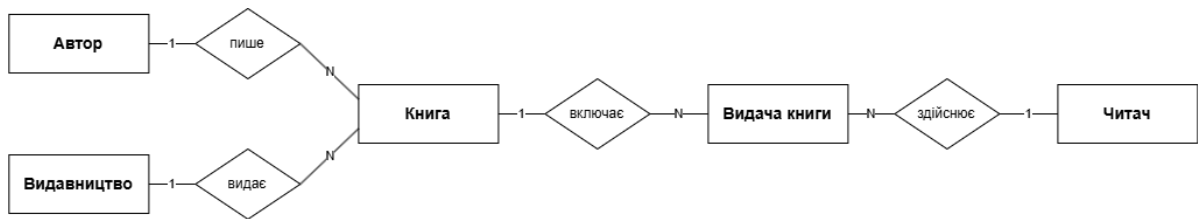
Рисунок 1.2 – Концептуальна ER-схема ПО «Бібліотека»
