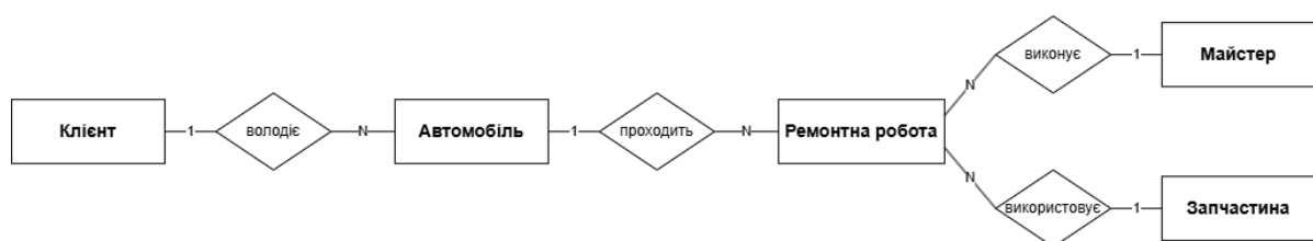
Рисунок 1.4 – Концептуальна ER-схема ПО «Автосалон / СТО»
