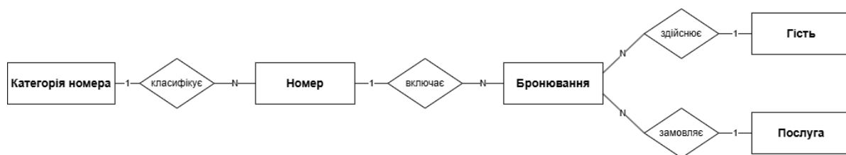
Рисунок 1.5 – Концептуальна ER-схема ПО «Готельний комплекс»
