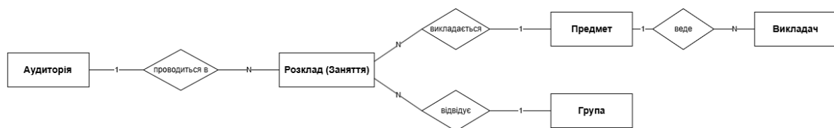
Рисунок 1.6 – Концептуальна ER-схема ПО «Університетський розклад»
