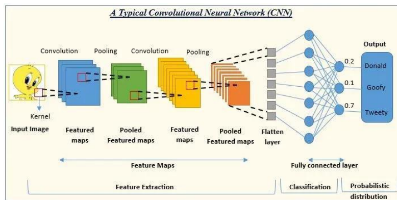
Hình 2.1 Kiến trúc cơ bản của mạng CNN
