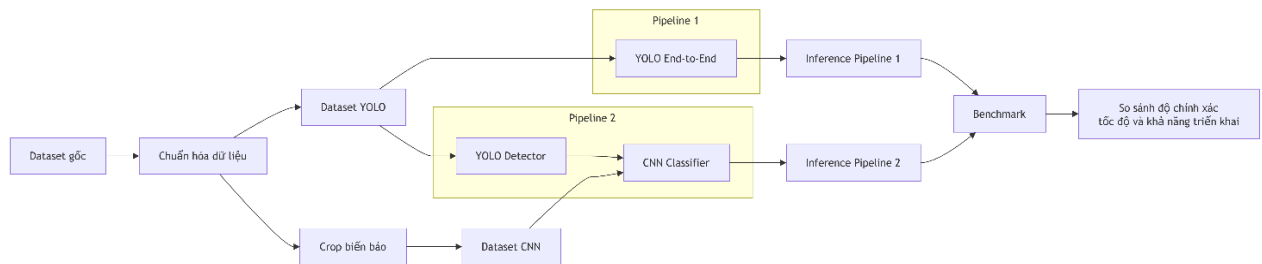
Hình 3.6 Cấu trúc 2 luồng kiểm thử
