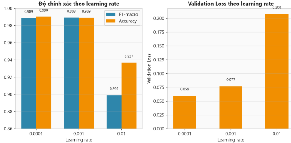
Hình 3.8 Kết quả ảnh hưởng của learning
