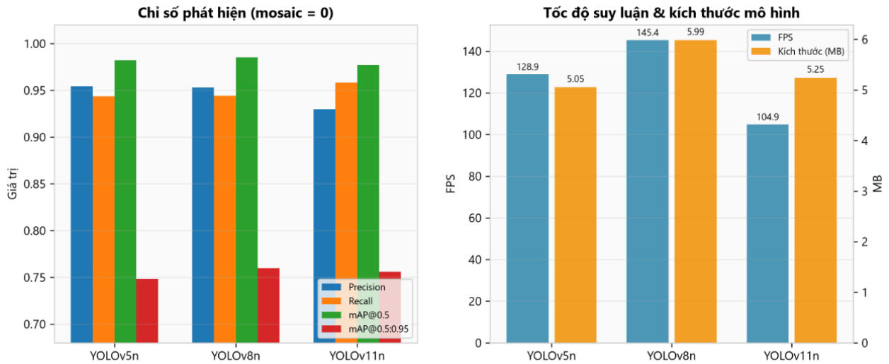
Hình 3.2 kết quả baseline của YOLO
