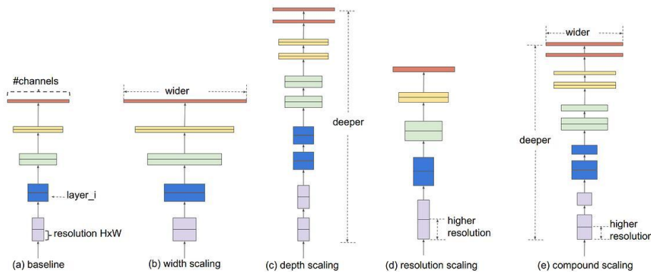
Hình 1.8 Kiến trúc EfficientNet
