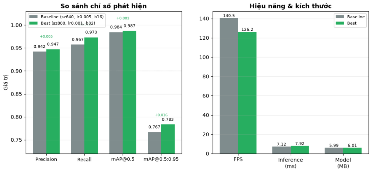
Hình 3.6 Kết quả so với baseline
