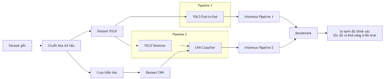
Hình 2.6 Cấu trúc 2 luồng kiểm thử
