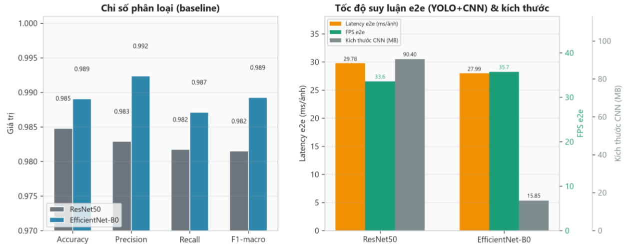
Hình 3.7 Kết quả baseline của CNN
