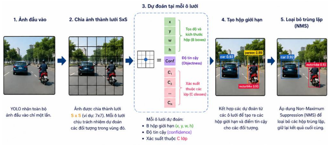
Hình 1.6 Nguyên lý hoạt động của YOLO
