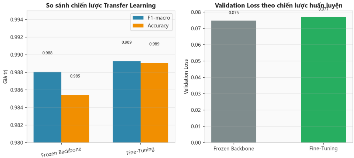
Hình 3.9 Ảnh hưởng của transfer learning
