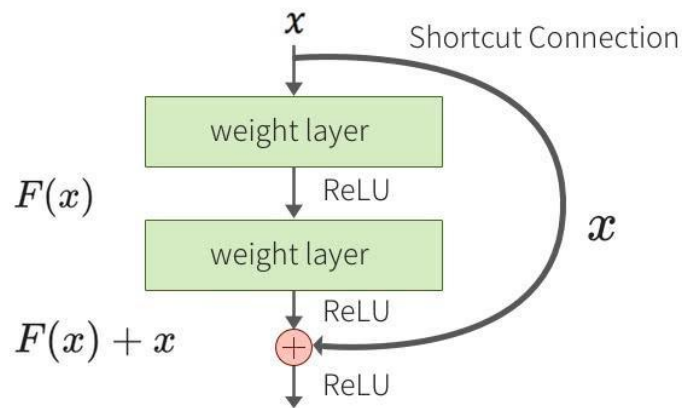
Hình 1.7 Kiến trúc mạng ResNet
