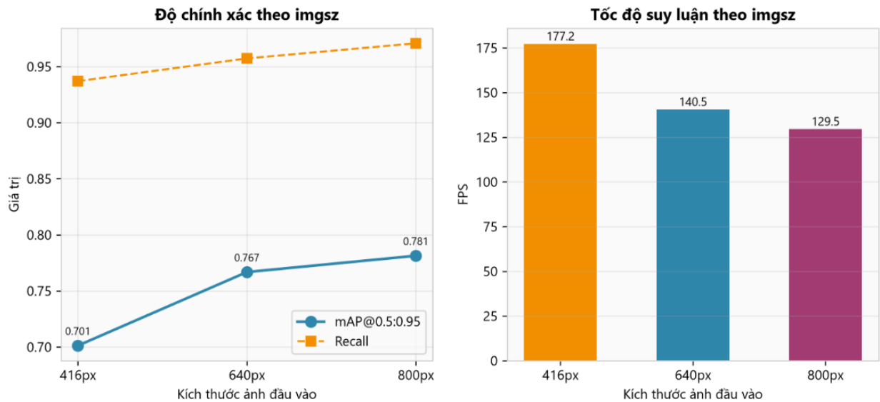
Hình 3.3 kết quả ảnh hưởng của imgsize
