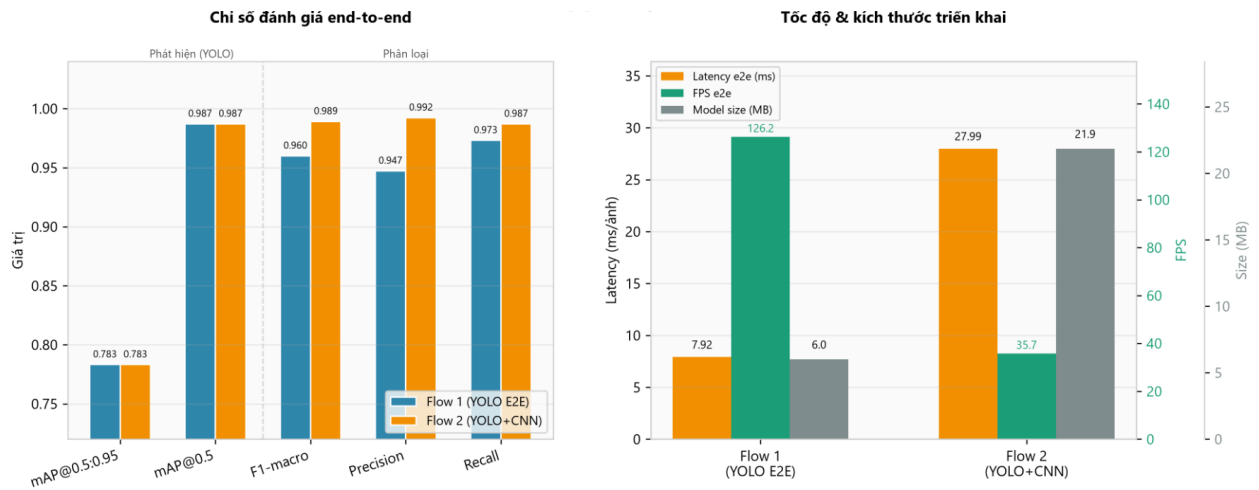
Hình 3.10 Kết quả đánh giá luồng CNN
