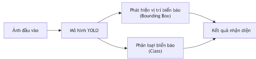
Hình 2.7 Luồng kiểm thử YOLO End-to-End
