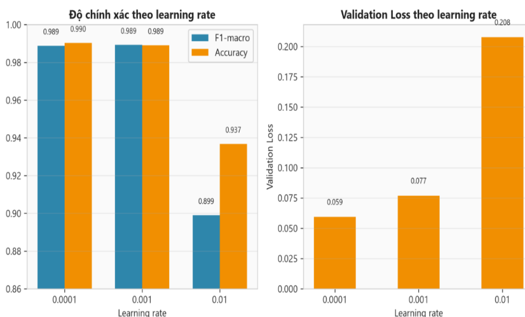
Hình 3.8 Kết quả ảnh hưởng của learning
