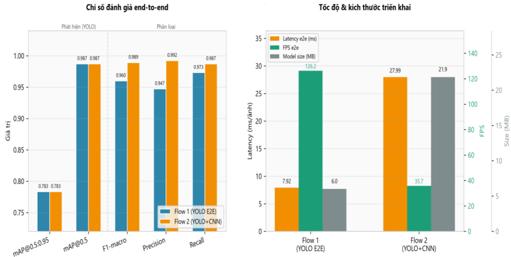
Hình 3.10 Kết quả đánh giá luồng CNN
