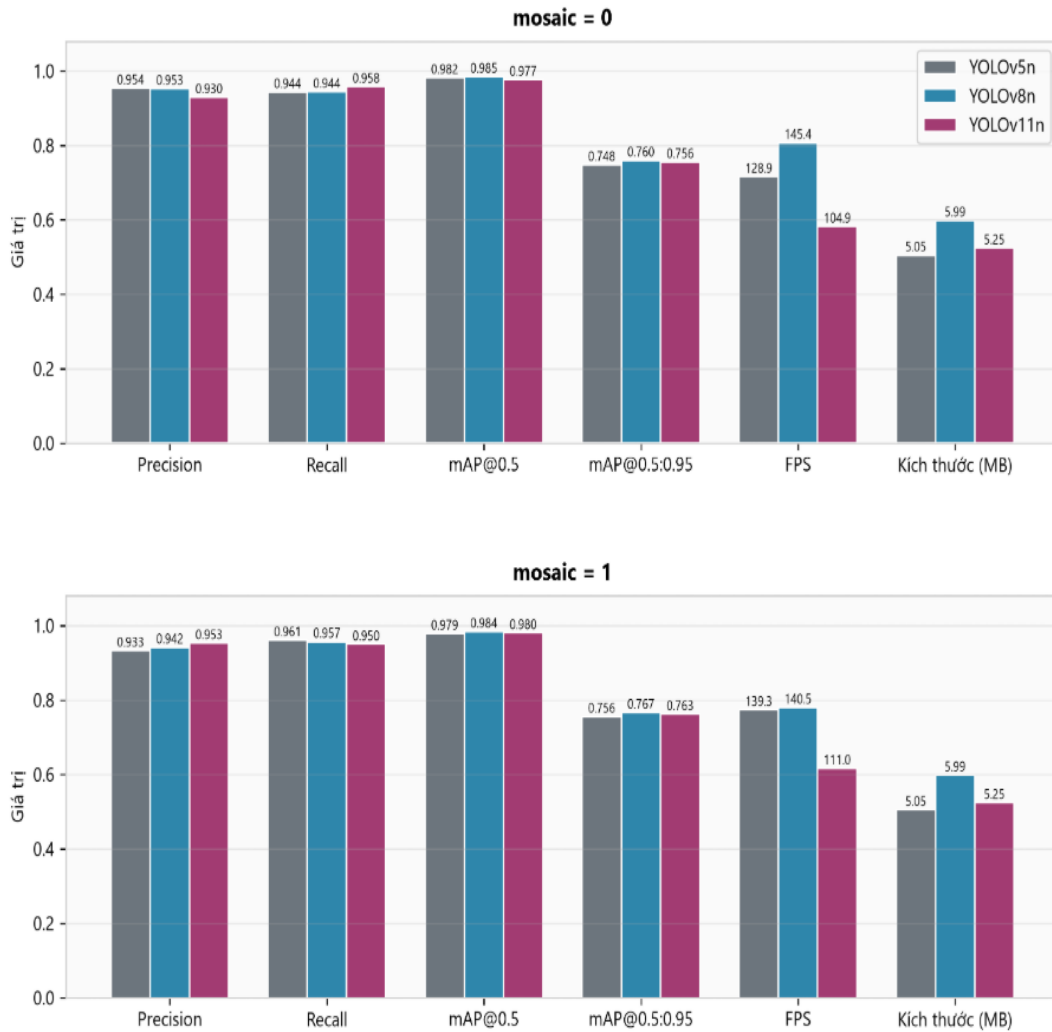
Hình 3.2 kết quả baseline của YOLO
