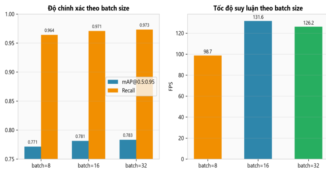
Hình 3.5 kết quả ảnh hưởng batchsize
