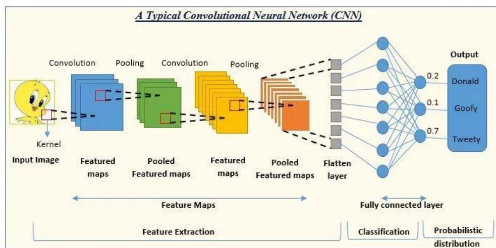
Hình 1.1 Kiến trúc cơ bản của mạng CNN
