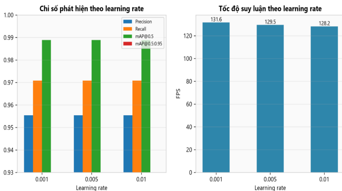
Hình 3.4 Kết quả ảnh hưởng của learning
