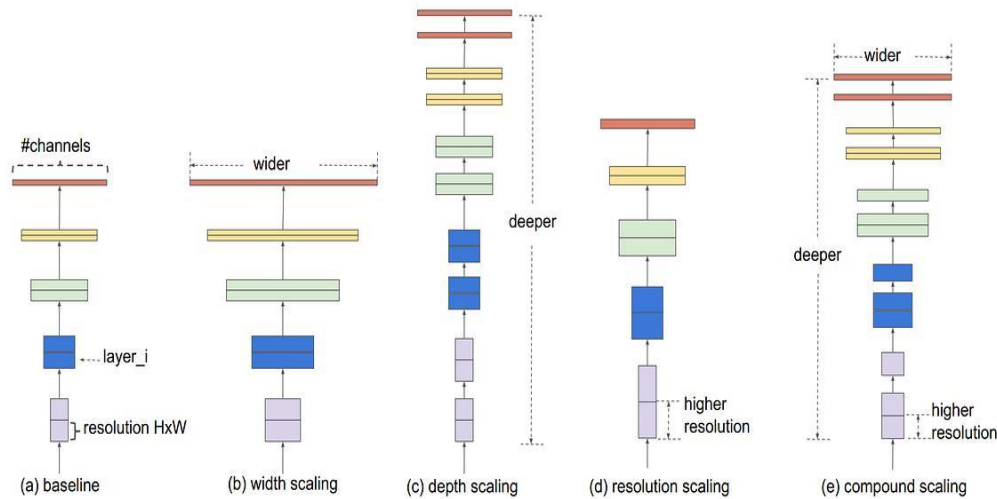
Hình 1.8 Kiến trúc EfficientNet
