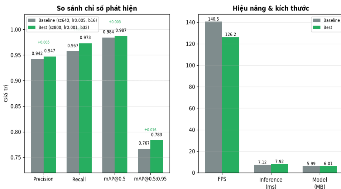
Hình 3.6 Kết quả so với baseline
