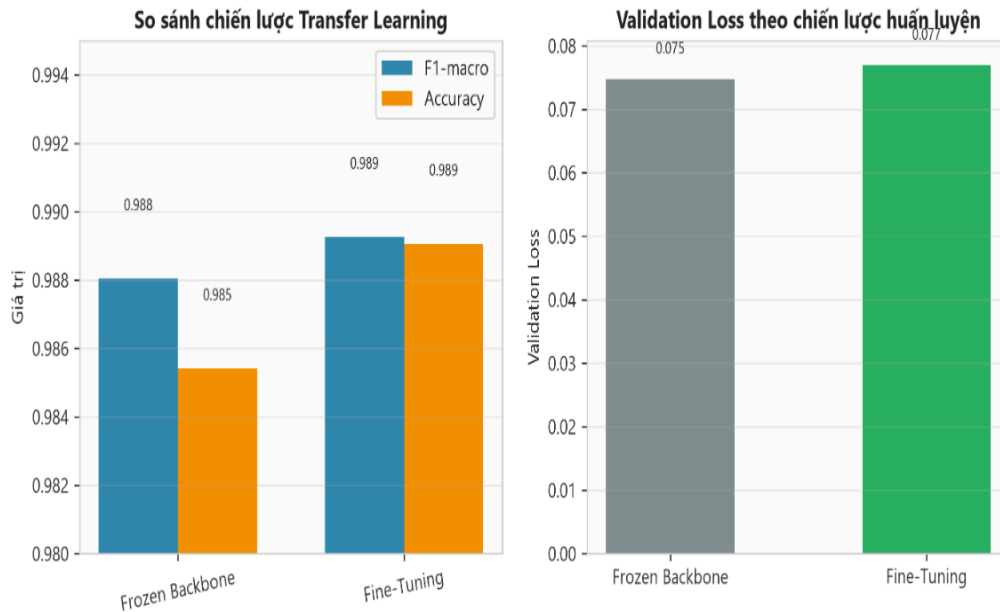
Hình 3.9 Ảnh hưởng của transfer learning
