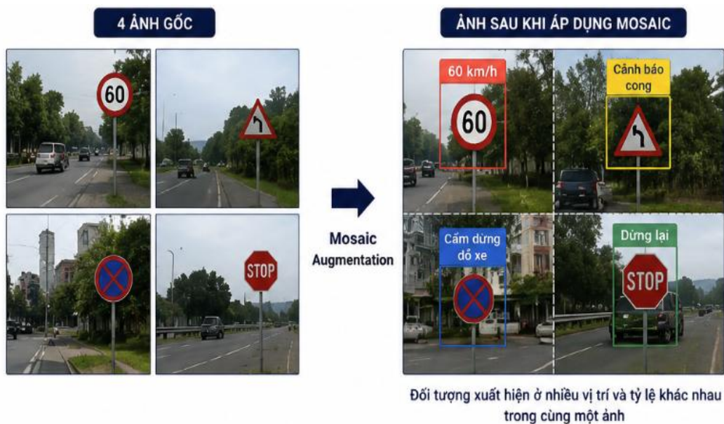
Hình 2.9 Kỹ thuật Mosaic
