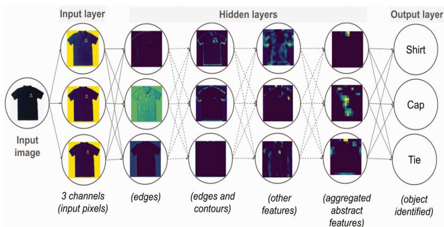
Hình 1.3 Cơ chế học đặc trưng phân cấp
