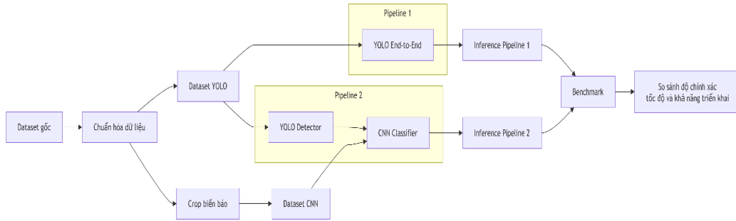
Hình 2.6 Cấu trúc 2 luồng kiểm thử
