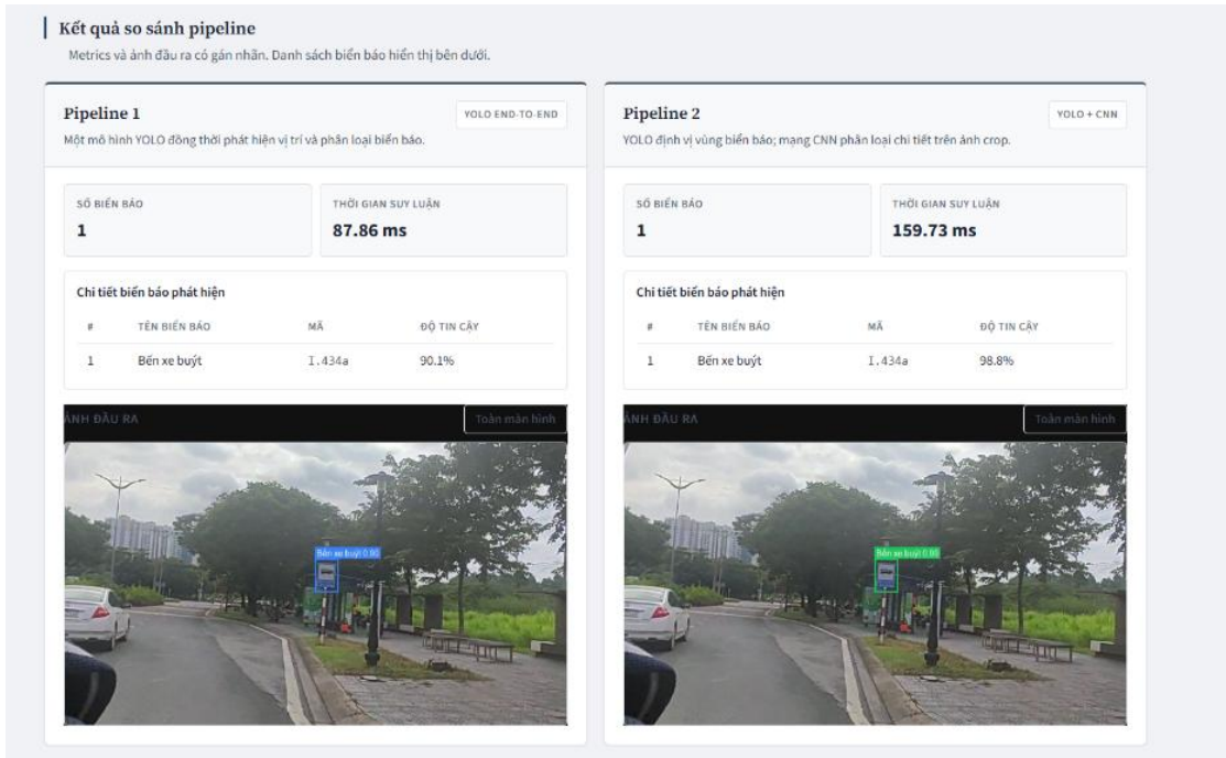
Hình 3.12 Giao diện nhận diện ảnh tĩnh
