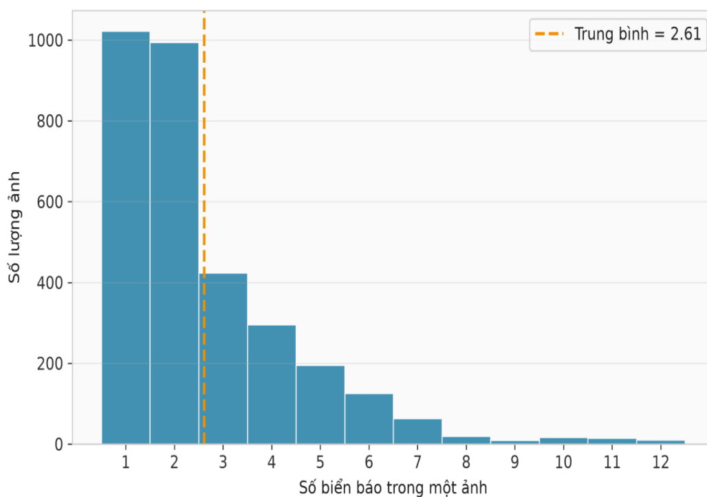
Hình 2.1 Trung bình biển báo mỗi ảnh
