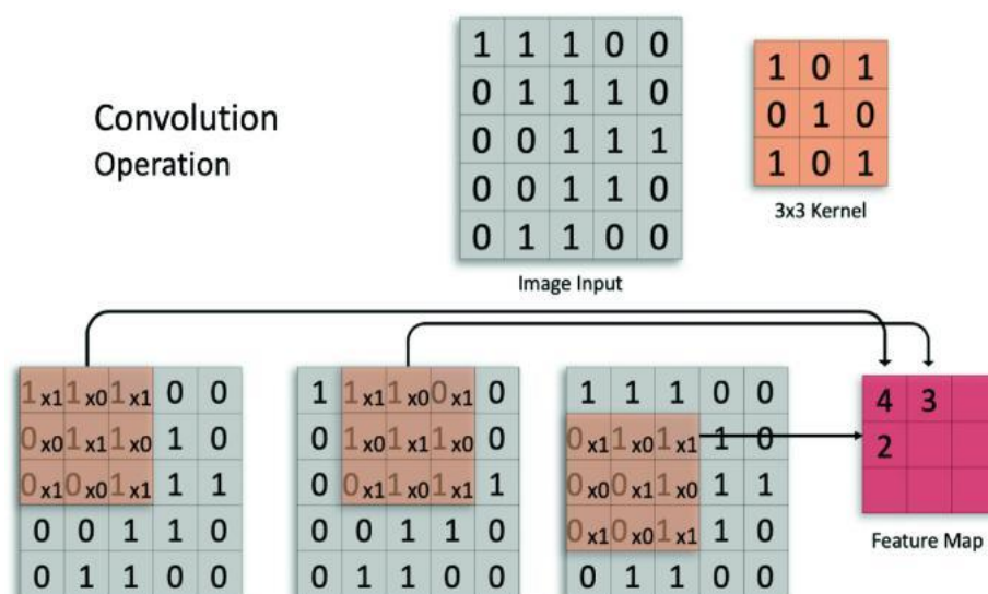
Hình 1.2 Minh họa quá trình tích chập
