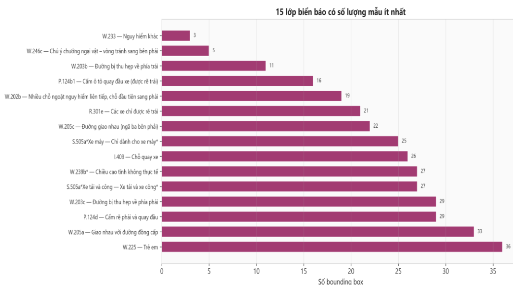
Hình 2.3 15 lớp có số mẫu ít nhất
