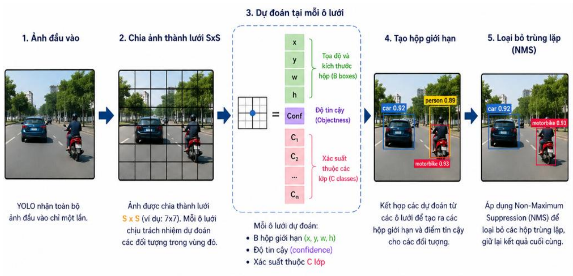
Hình 1.6 Nguyên lý hoạt động của YOLO
