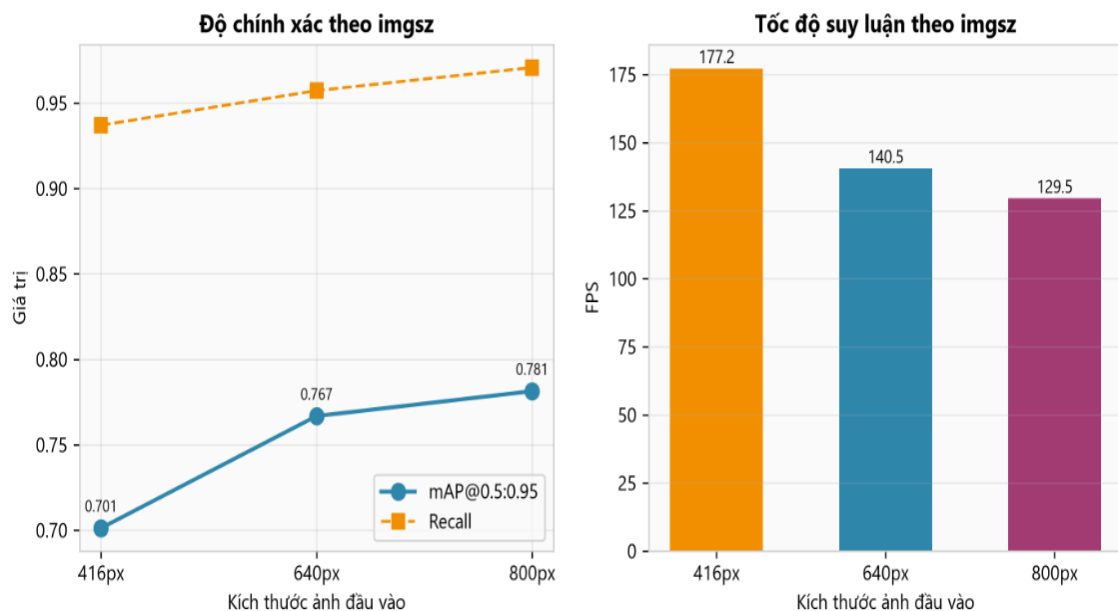
Hình 3.3 Kết quả ảnh hưởng của imgsize
