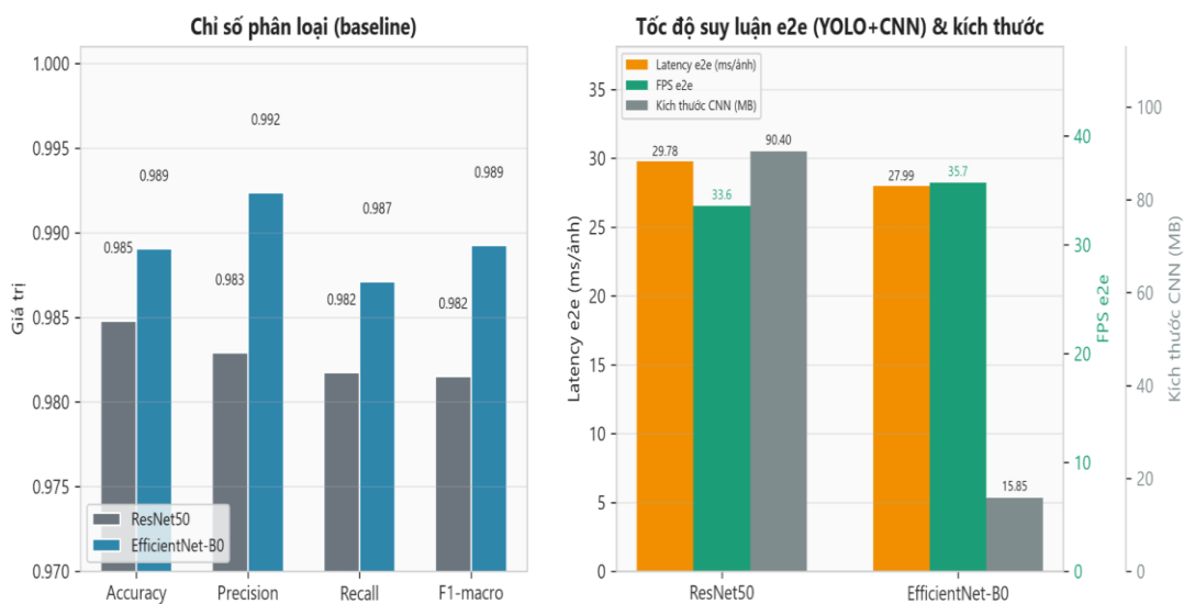
Hình 3.7 Kết quả baseline của CNN
