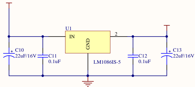
5V供外设转换电路
