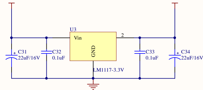
3.3V转换电路
