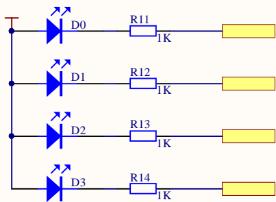
LED模块
