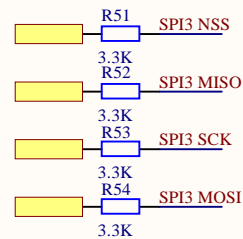
TF卡接口外围电路
