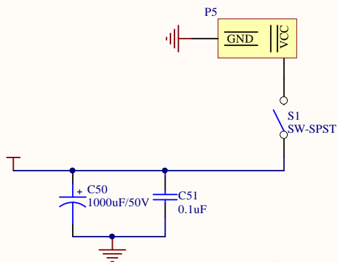
电源输入电路
