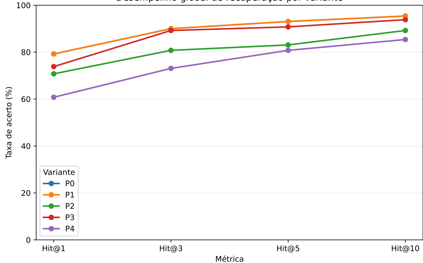
Desempenho global de recuperação por variante
