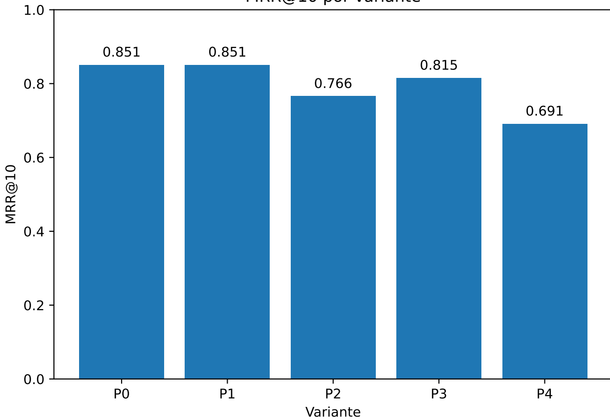
MRR@10 por variante
