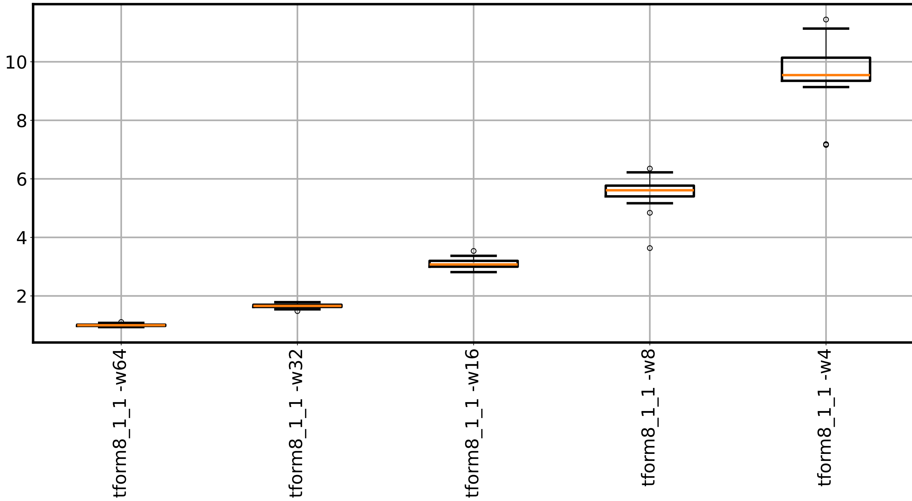
sort-small
