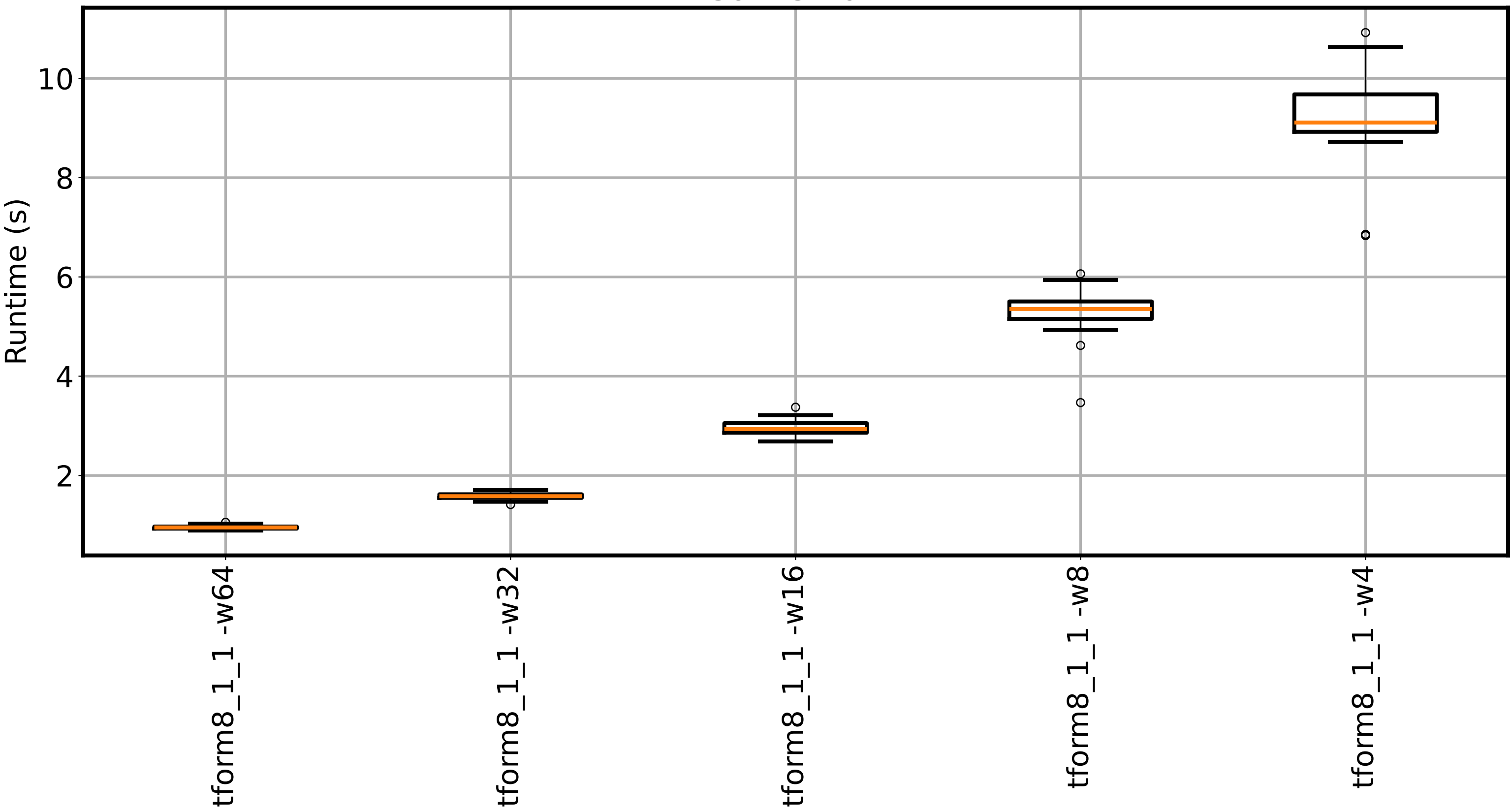
sort-small
