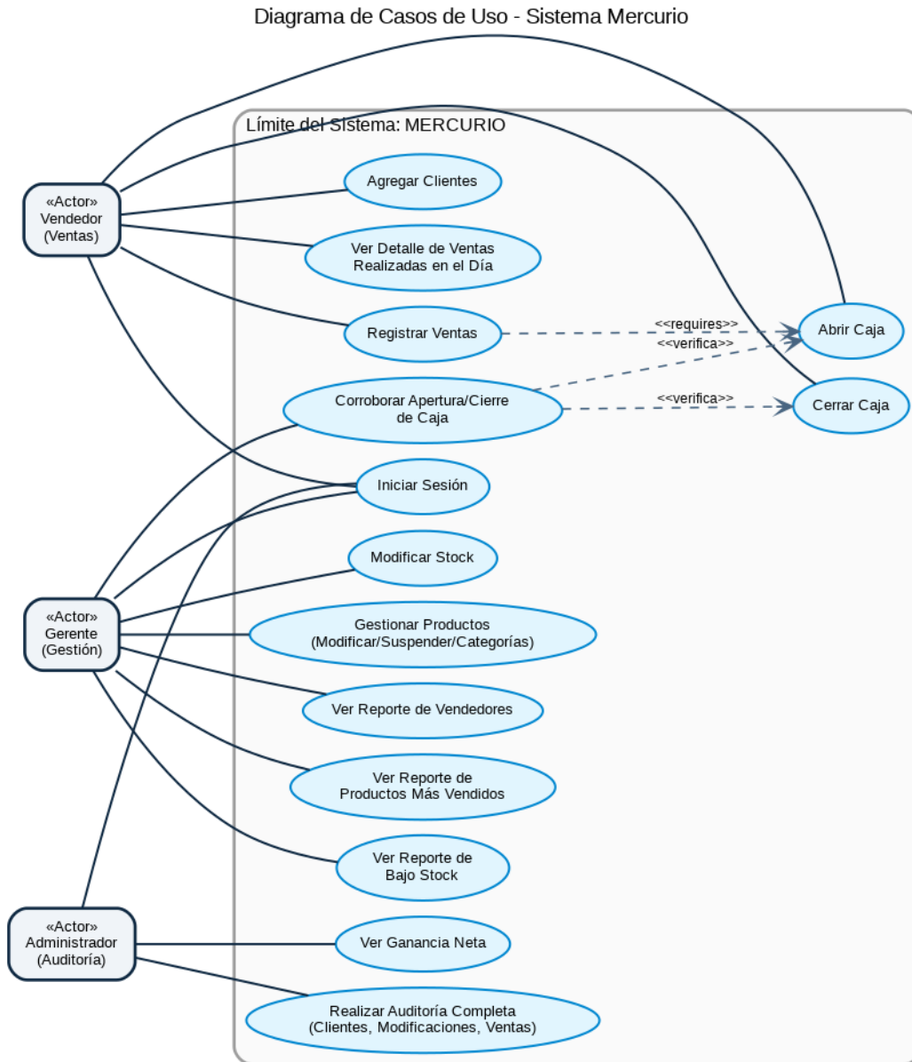
Figura 1: Diagrama de Casos de Uso UML para el Sistema Mercurio
