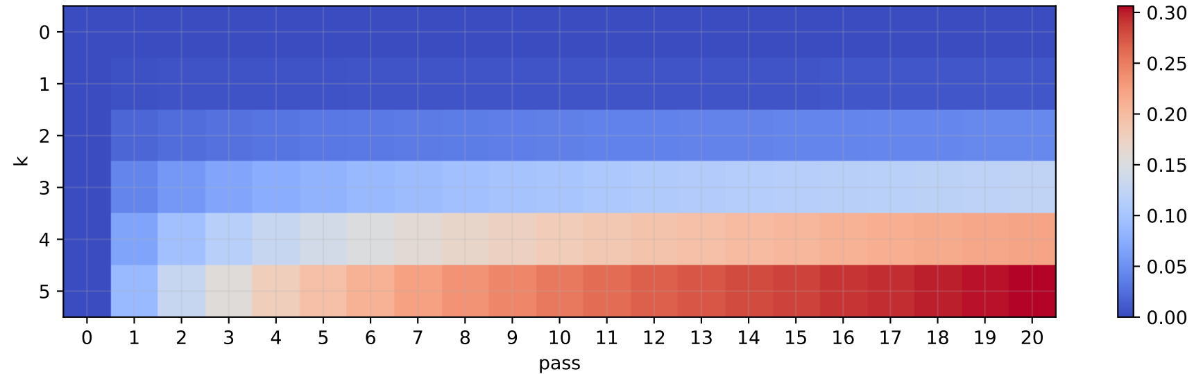
PokerHand: Validation NLL - train NLL
