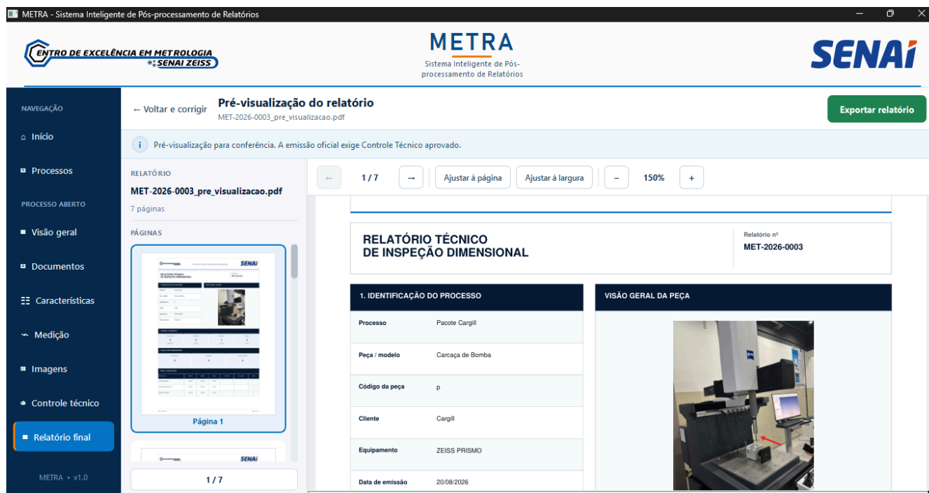
Figura 13 - Pré-visualização do relatório.
