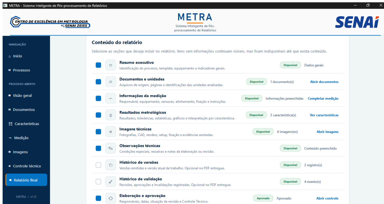
Figura 12 - Seleção das seções do relatório.
