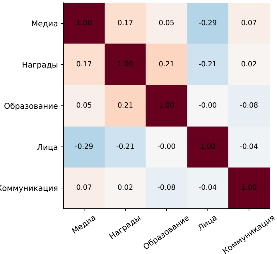
Все менеджеры: Spearman, n=64
