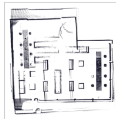
RKO-LIO
