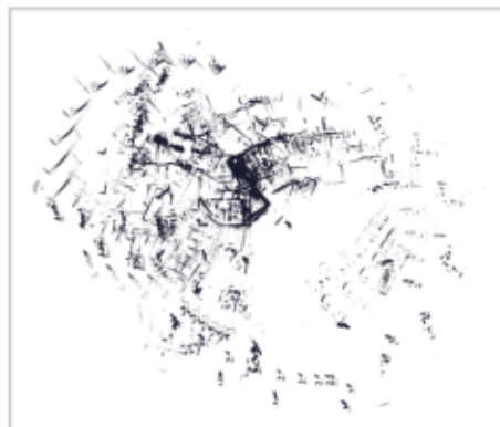
LIO-SAM
