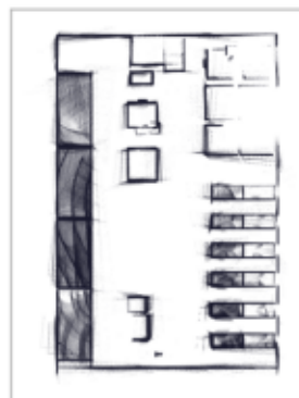
LIO-SAM
