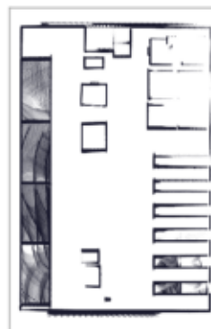
RKO-LIO
