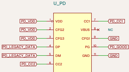
CH224K
