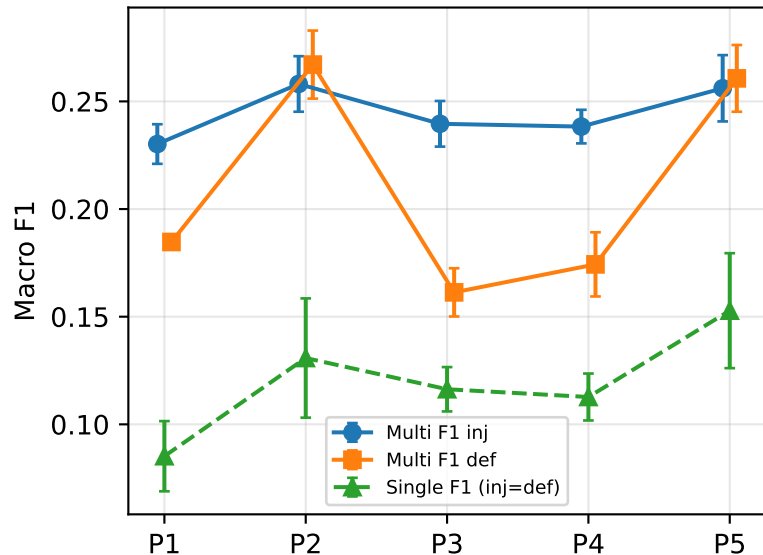
F1 under injection (mean \pm std)
