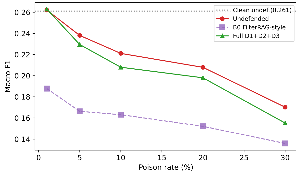
F1 vs poison rate
