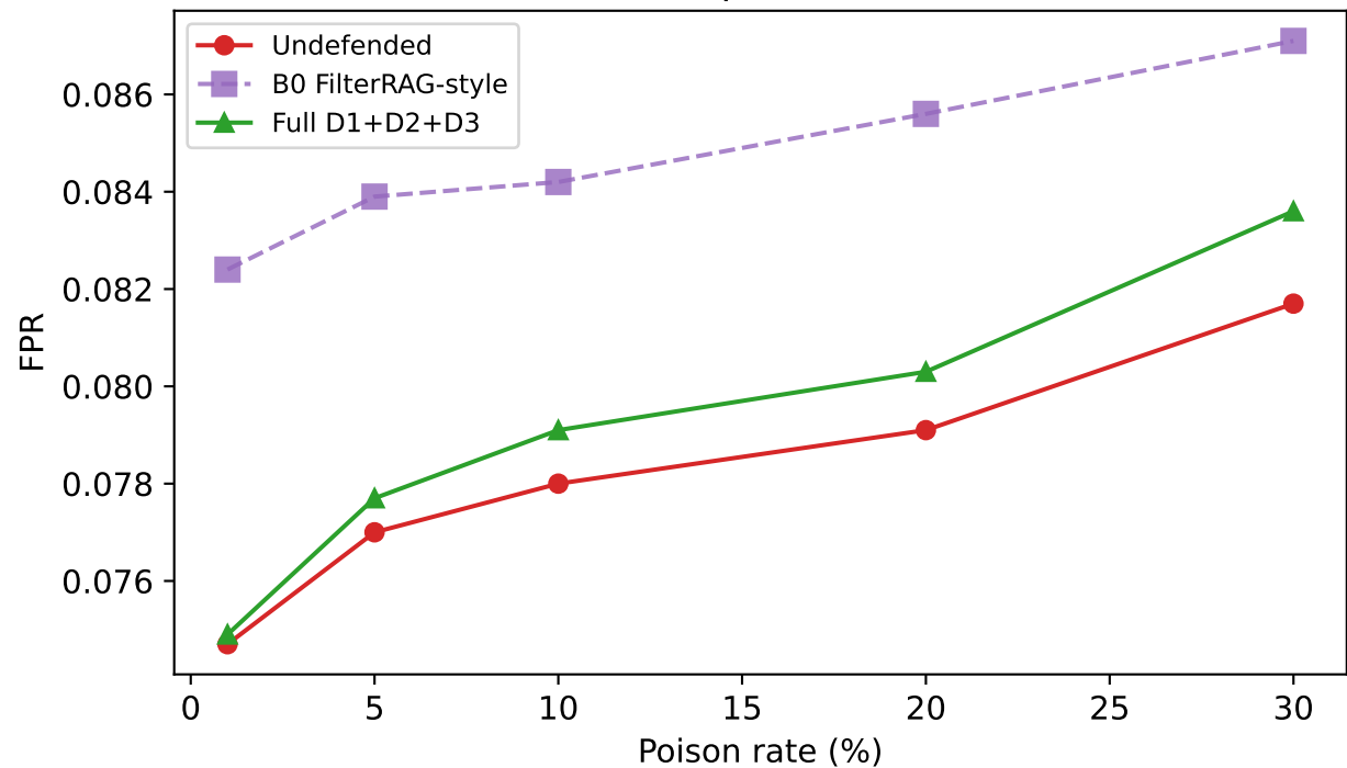
FPR vs poison rate
