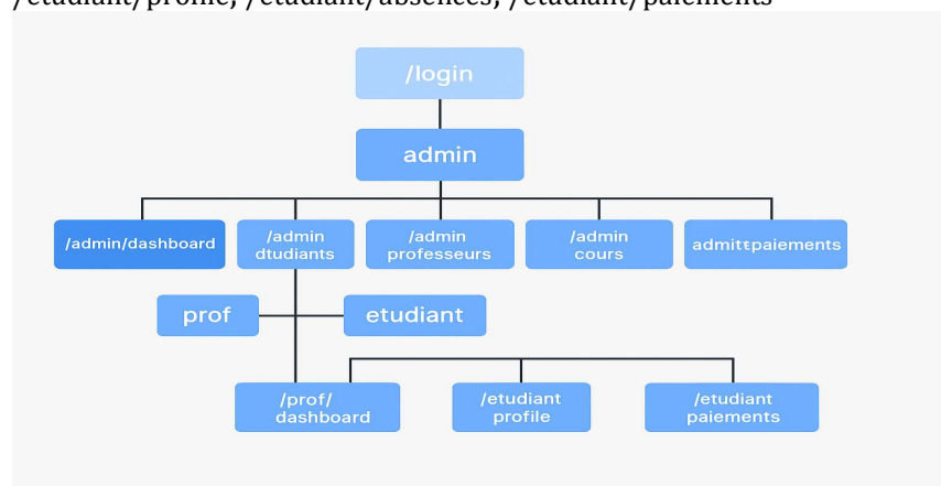
❏ (Figure 14 : Arborescence des routes principales)
