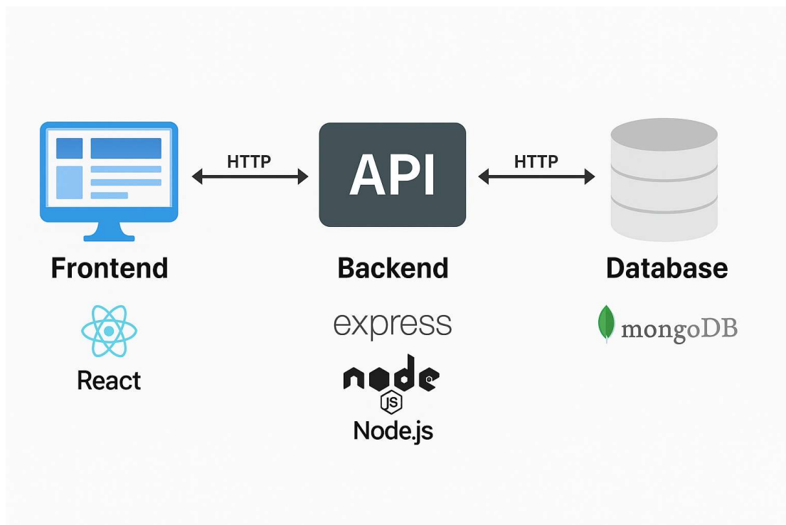
2 (Figure 8 : Schéma technique des flux – React ↔ API ↔ MongoDB)
