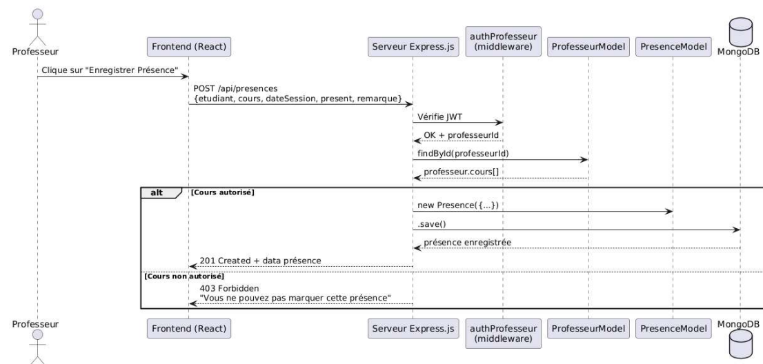
Figure 11 : Diagramme de séquence – marquage de présence
