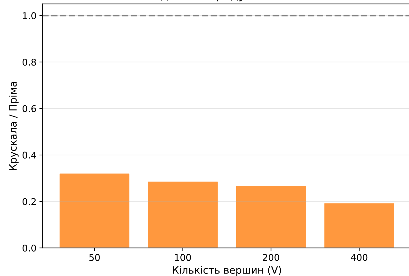
Відносна продуктивність
