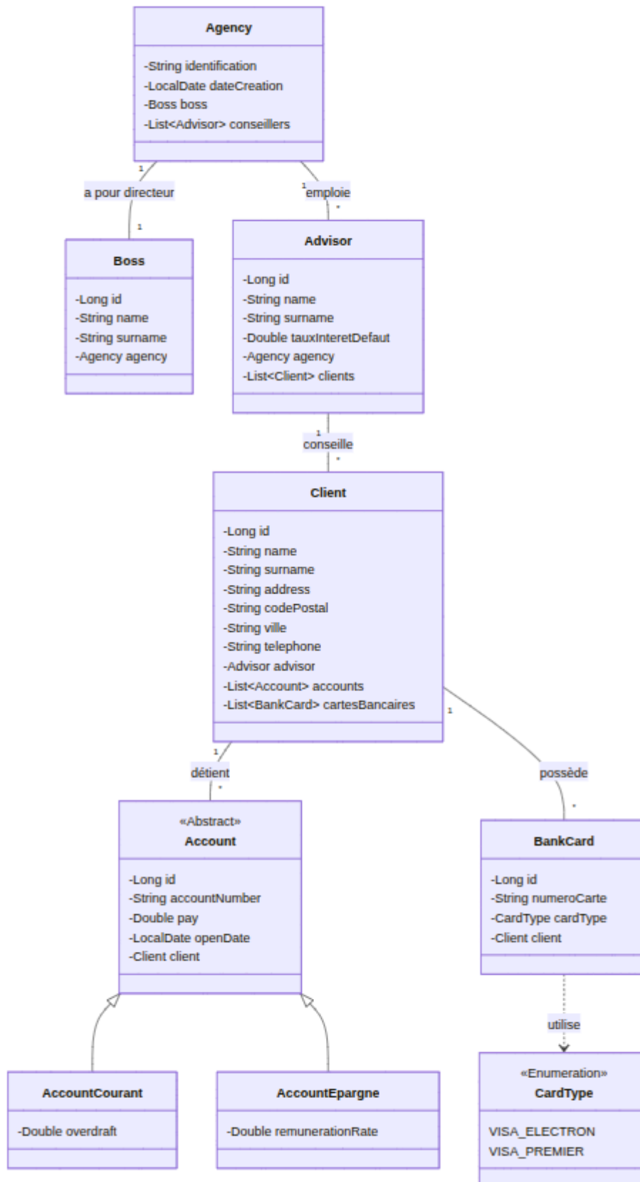
Schéma UML de la DB :
