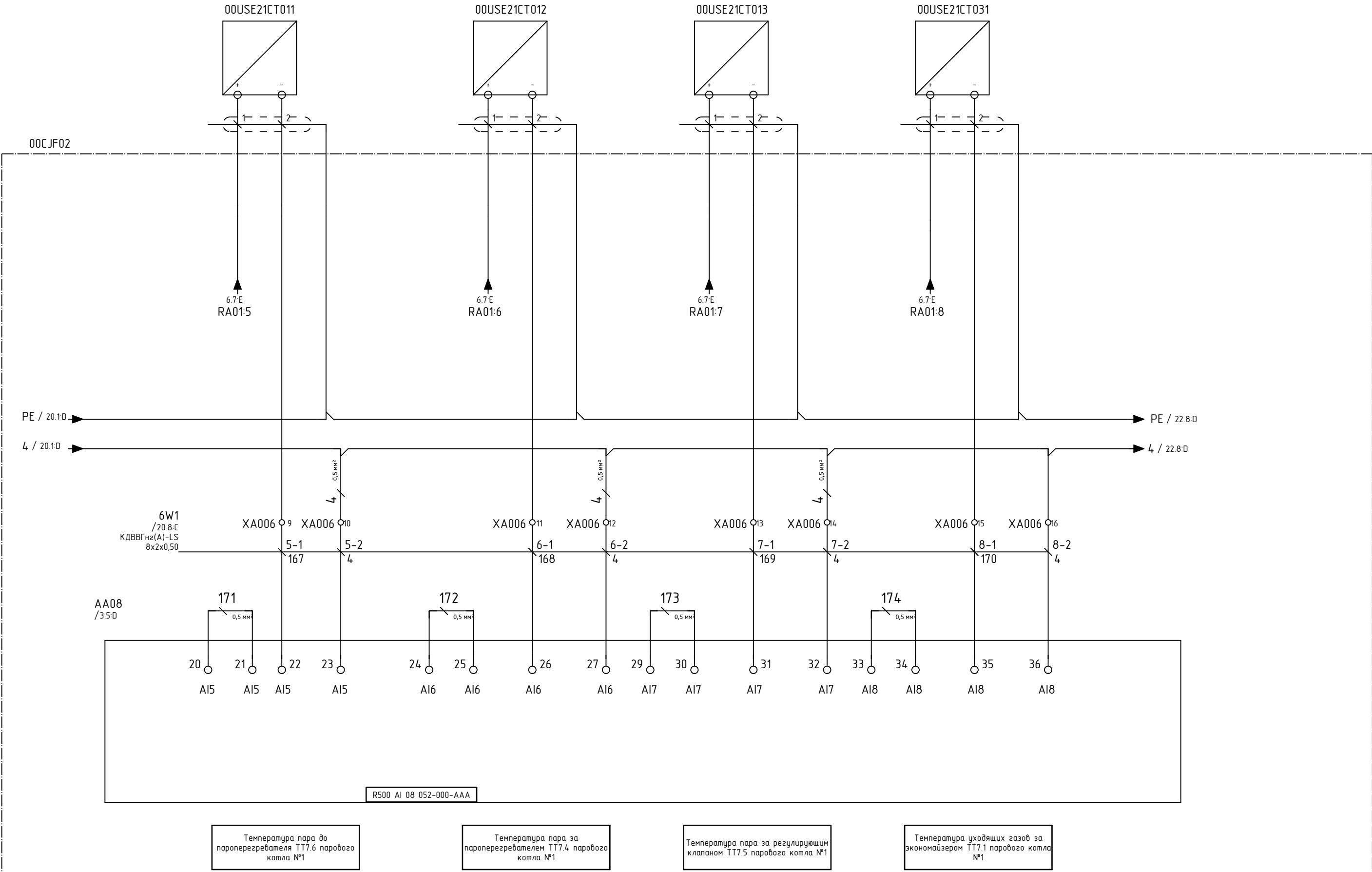
Схема соединения модуля AA08
