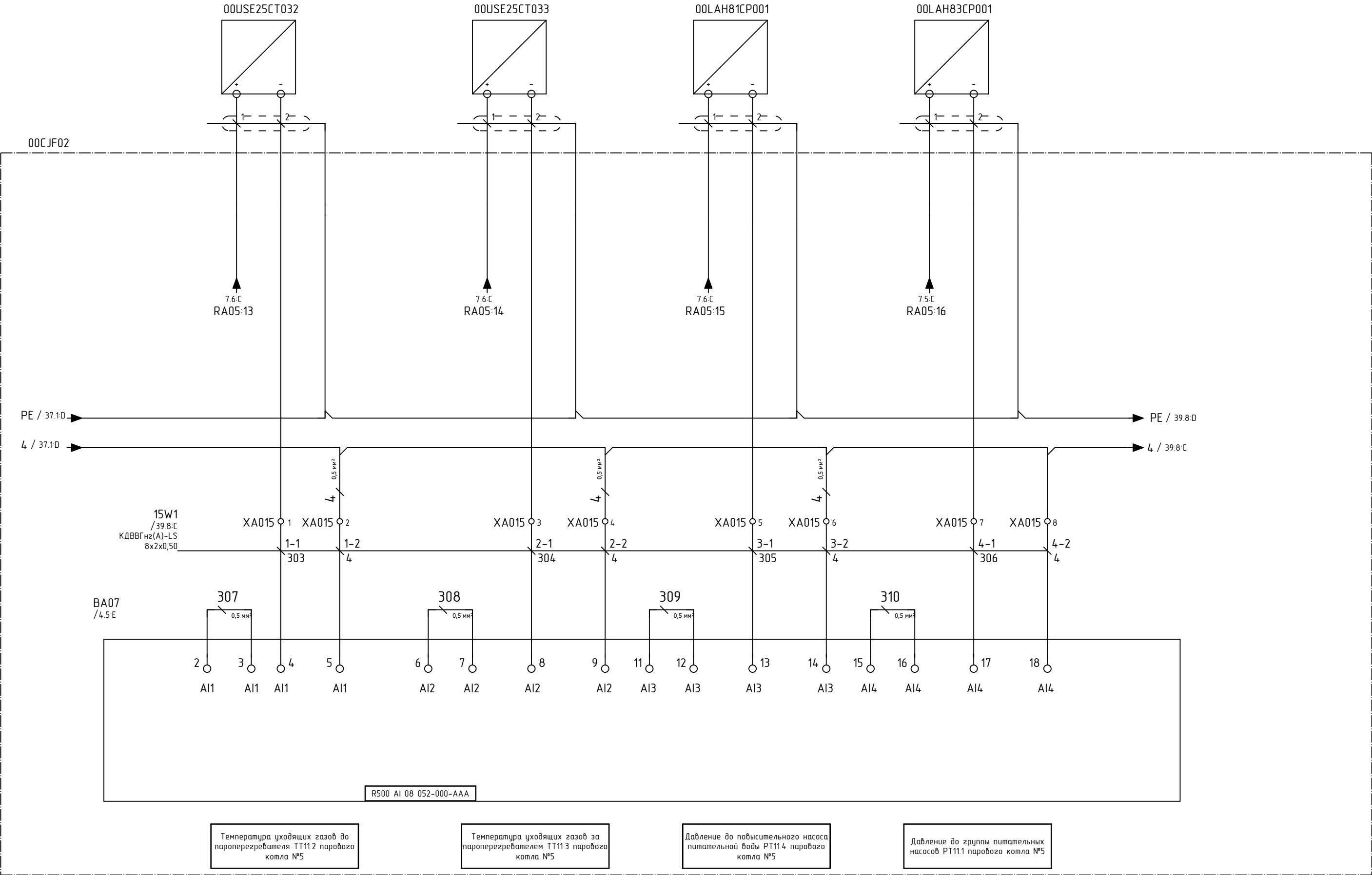
Схема соединения модуля ВА07
