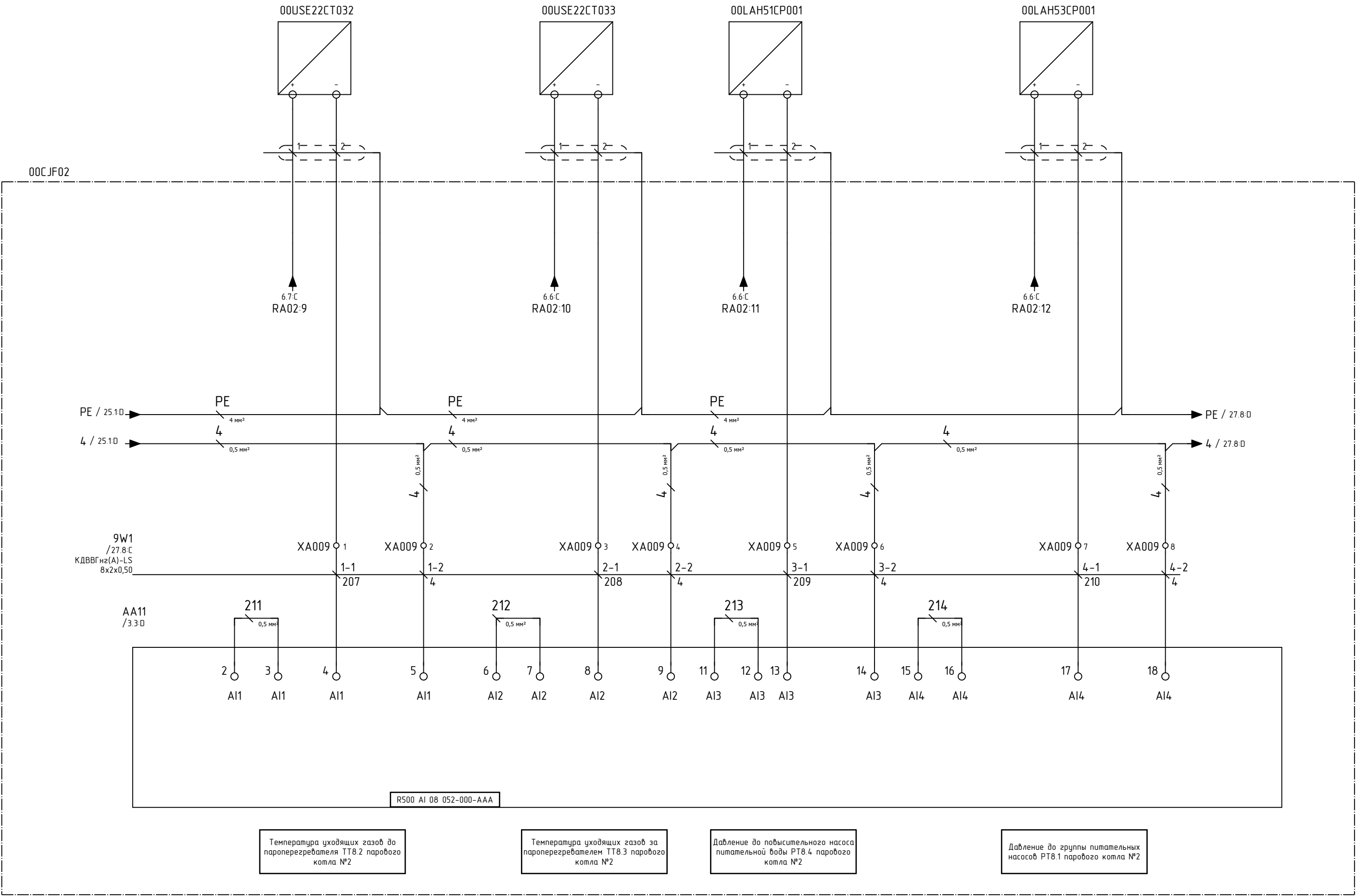
Схема соединения модуля AA11
