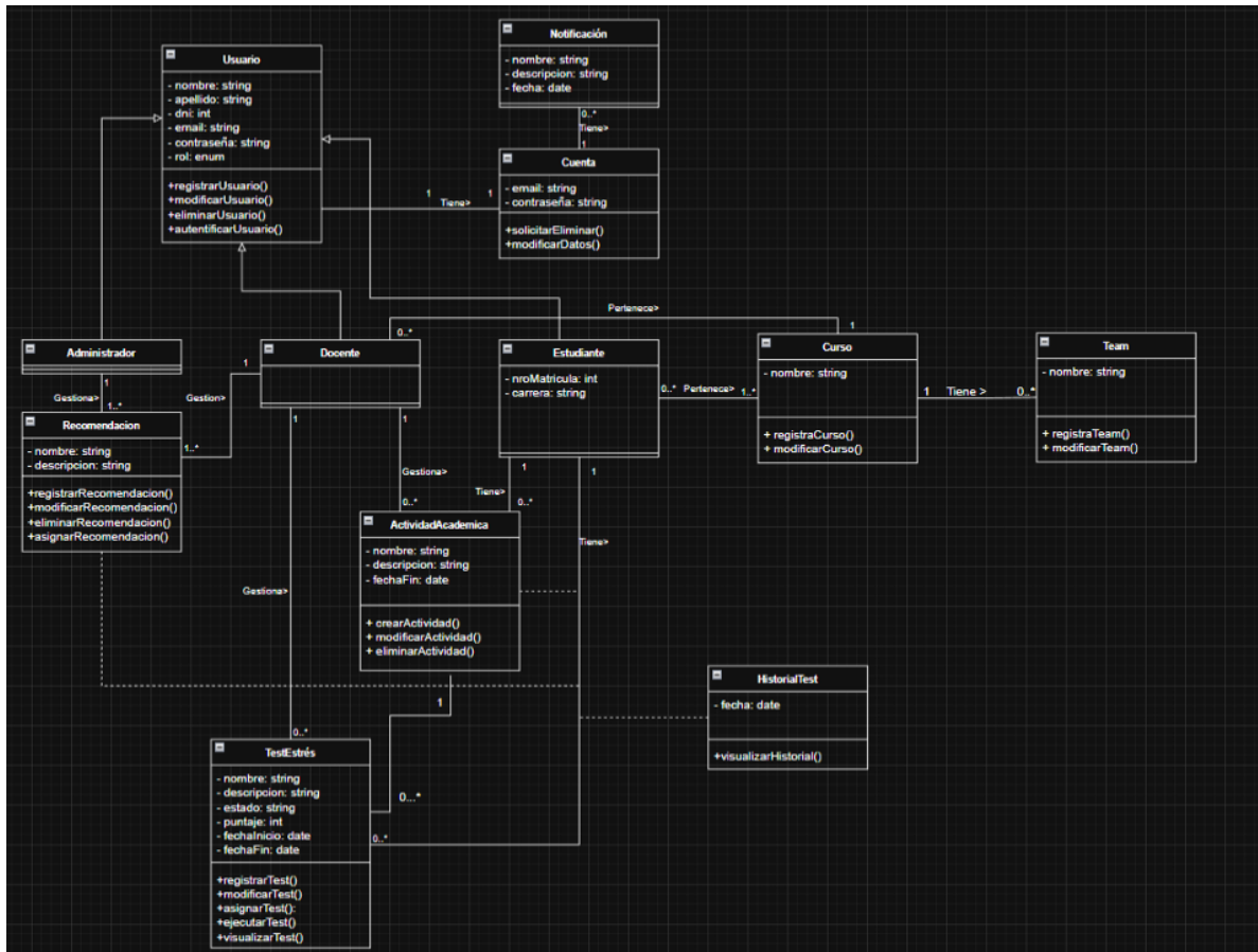
Figure 4: Diagrama de Clases (Nivel 4)
