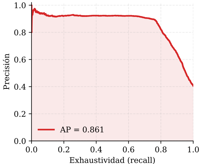
Curva Precisión-Exhaustividad
