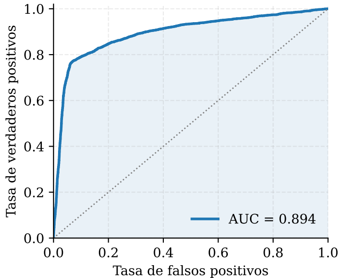
Curva ROC
