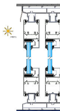
Corte Horizontal
