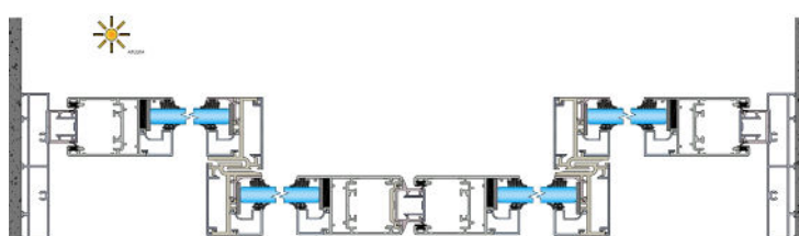
Corte Horizontal
