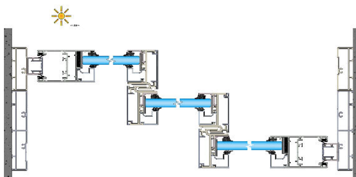
Corte Horizontal
