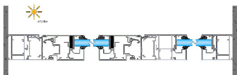
Corte Horizontal
