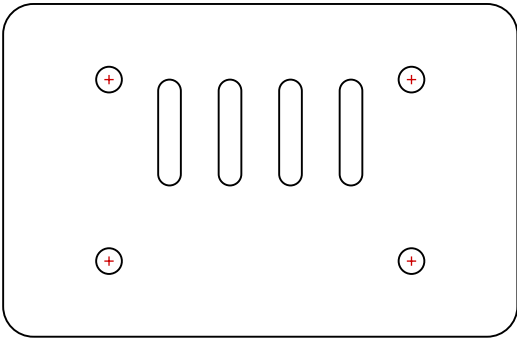
A2 Badan kamera - TUTUP belakang [Aluminium 2 mm] 68 x 44 mm
