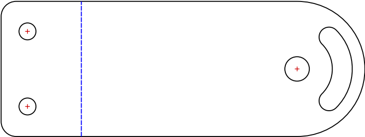
S3 Lengan KIRI [Baja 3 mm] 97 x 36 mm
