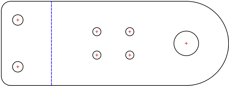
S4 Lengan KANAN [Baja 3 mm] 97 x 36 mm
