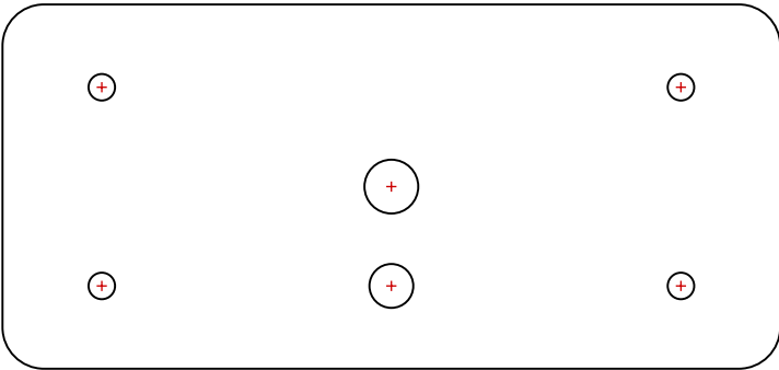
S1 Plat sisi KIRI badan kamera [Baja 3 mm] 94 x 44 mm
