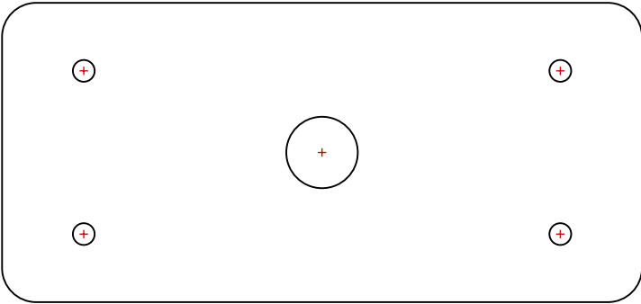
S2 Plat sisi KANAN badan kamera [Baja 3 mm] 94 x 44 mm
