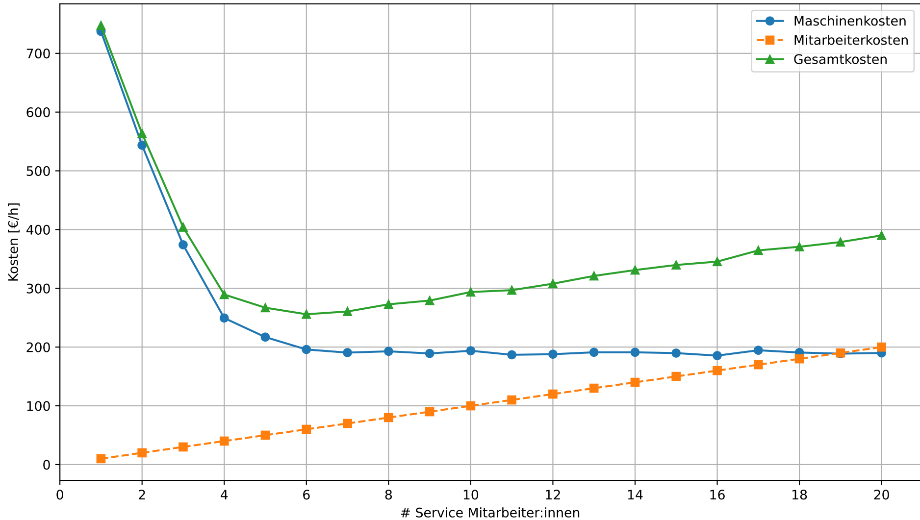
Kosten: 19 Maschine(n)
