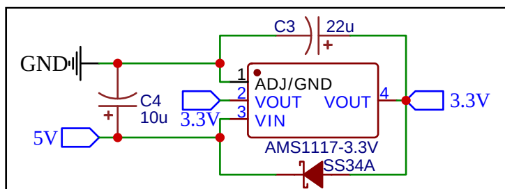
REGULADOR 3.3V
