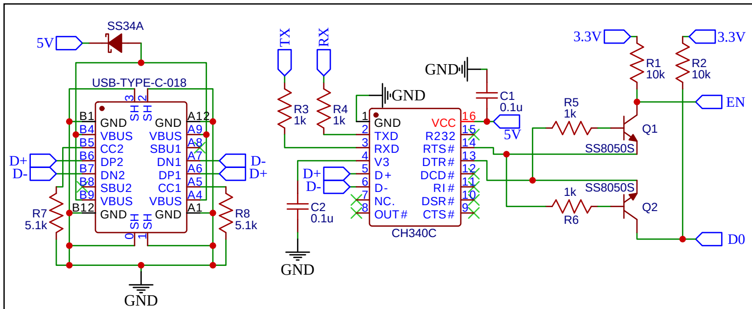
PROGRAMADOR POR USBC CH340
