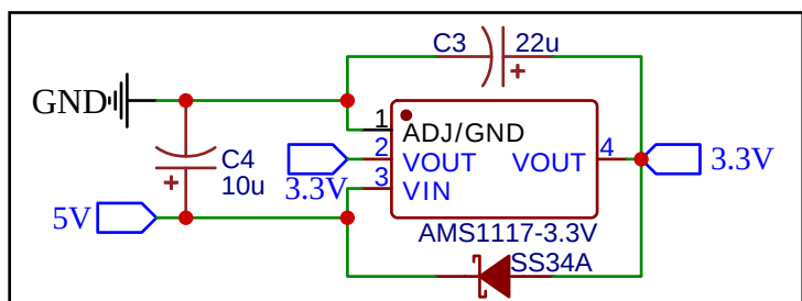
REGULADOR 3.3V
