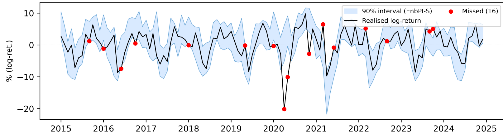
EnbPI-S
