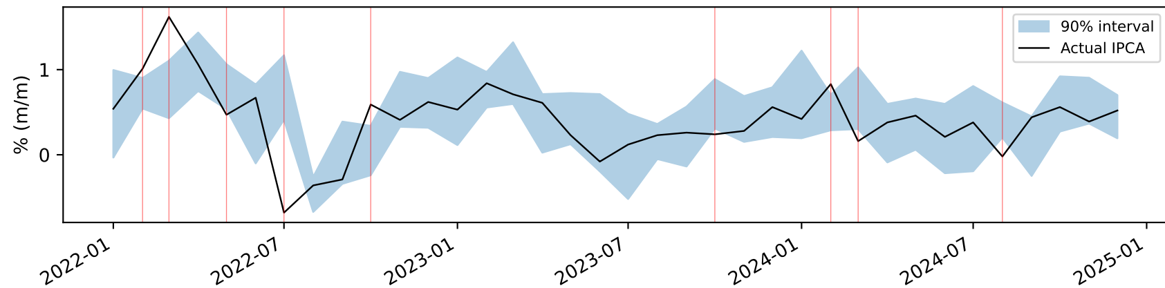
EnbPI-S
