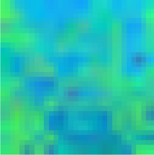
vit 14×14 grid
