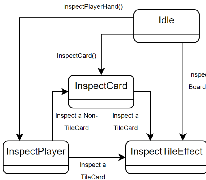
Figura 4.5: Transição de estado da Interface do Jogo para inspecionar elementos na mão do jogador ou no tabuleiro
