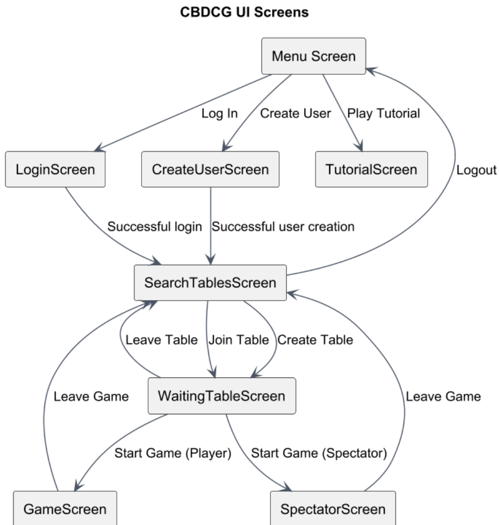
Figura 4.3: Transição de estados do Cliente
