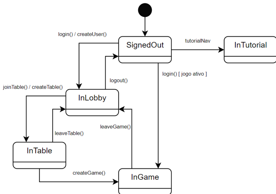
Figura 4.2: Transição de estados do Cliente
