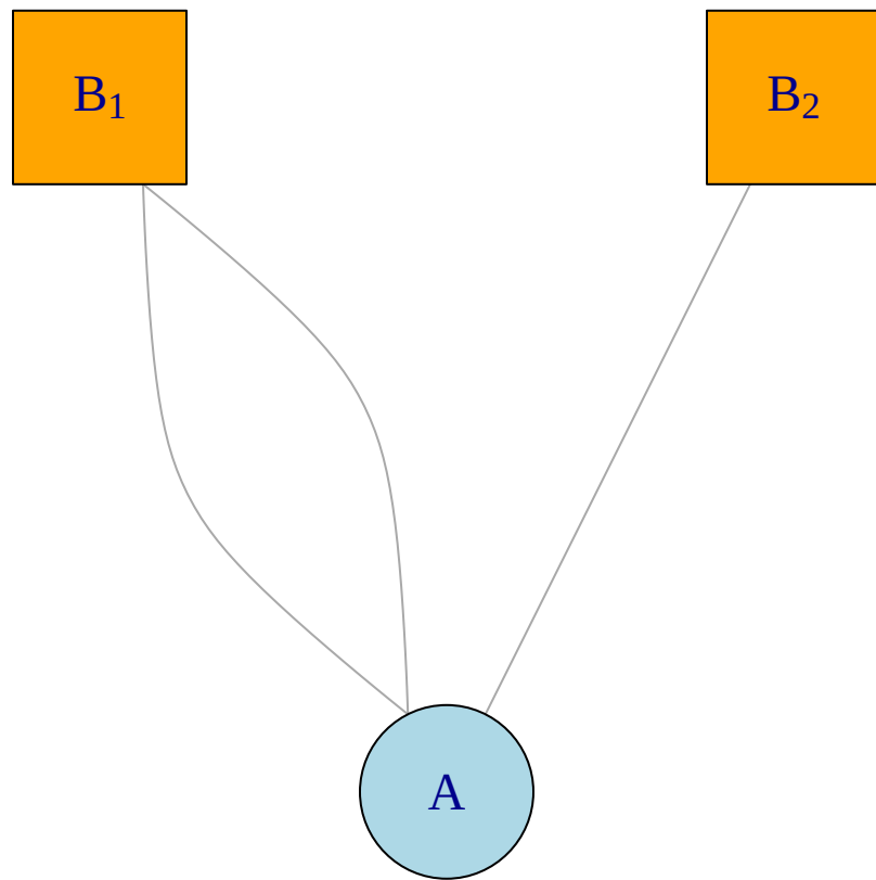
Weighted Bipartite
