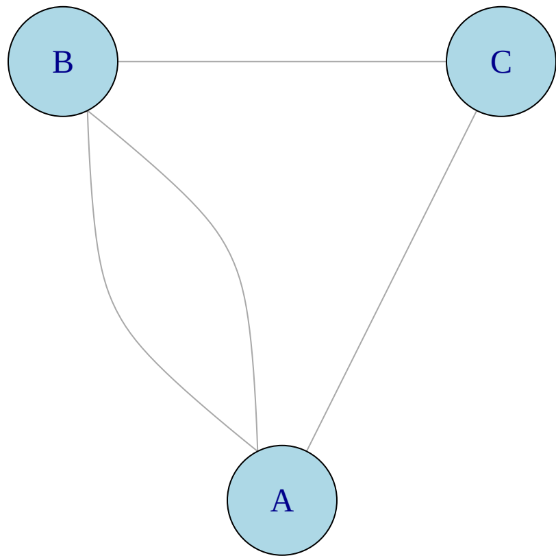
Unipartite
